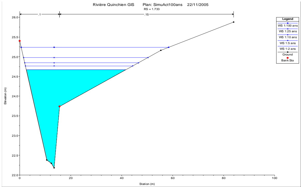
C-7a. Niveaux calculés avec le bassin actuel au ch 1+733
