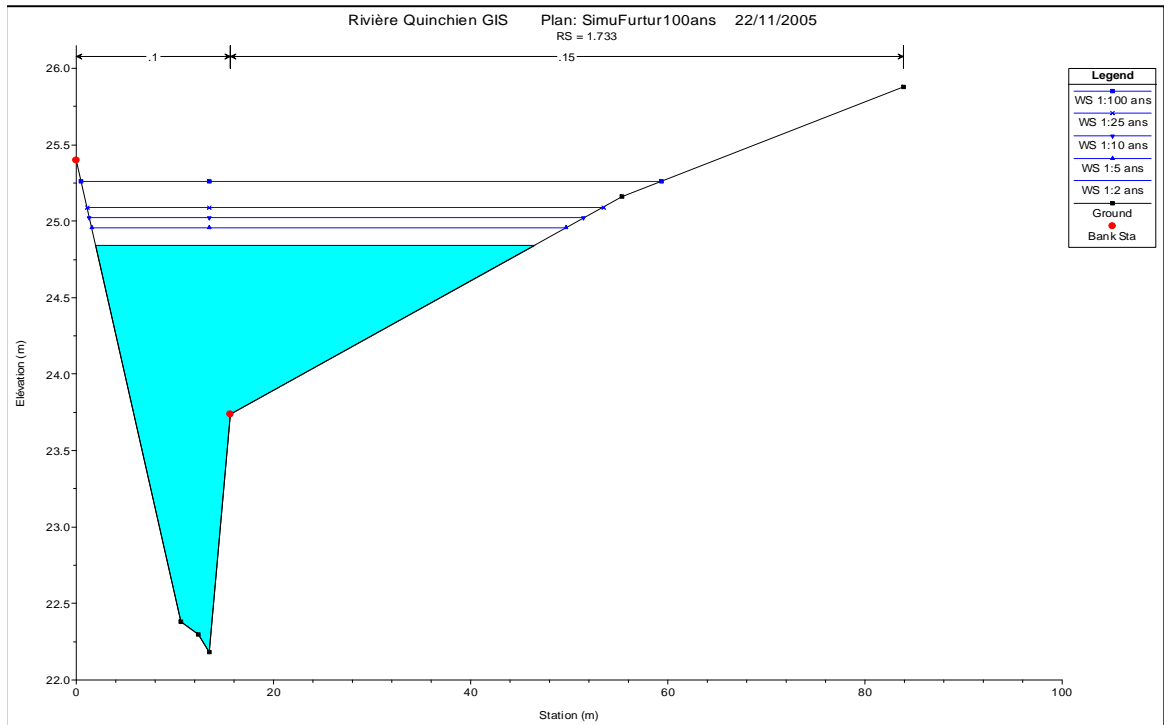
C-7b. Niveaux calculés avec le bassin futur au ch 1+733
