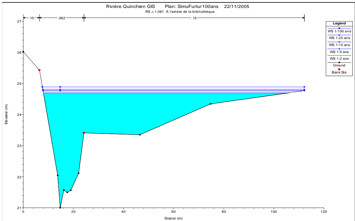
C-1b. Niveaux calculés avec le bassin futur au ch 1+061
