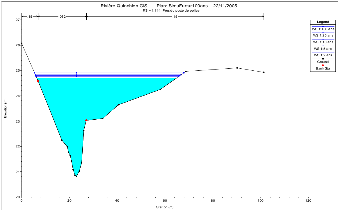
C-2b. Niveaux calculés avec le bassin futur au ch 1+114
