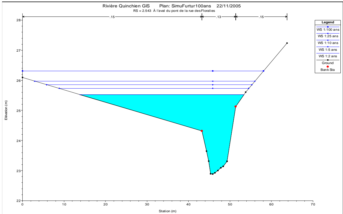
C-8b. Niveaux calculés avec le bassin futur au ch 2+543
