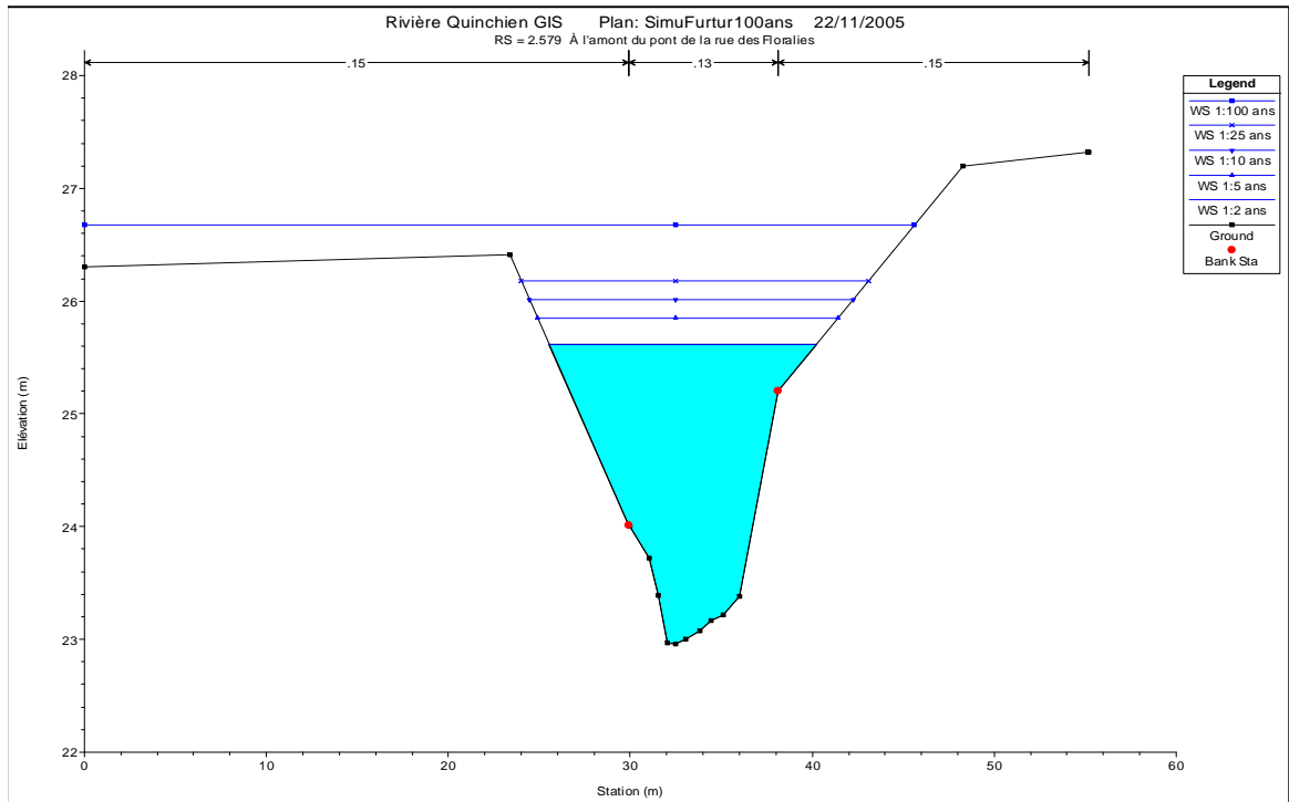
C-9b. Niveaux calculés avec le bassin actuel au ch 2+579
