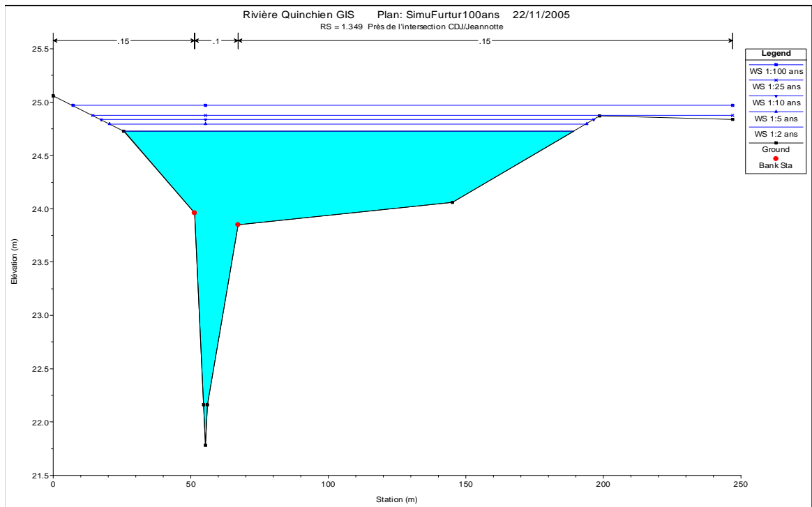
C-4b. Niveaux calculés avec le bassin futur au ch 1+349
