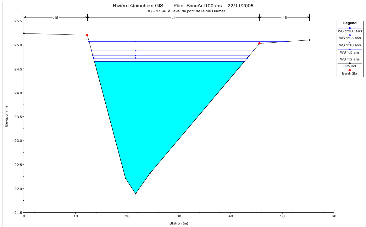
C-5a. Niveaux calculés avec le bassin actuel au ch 1+594
