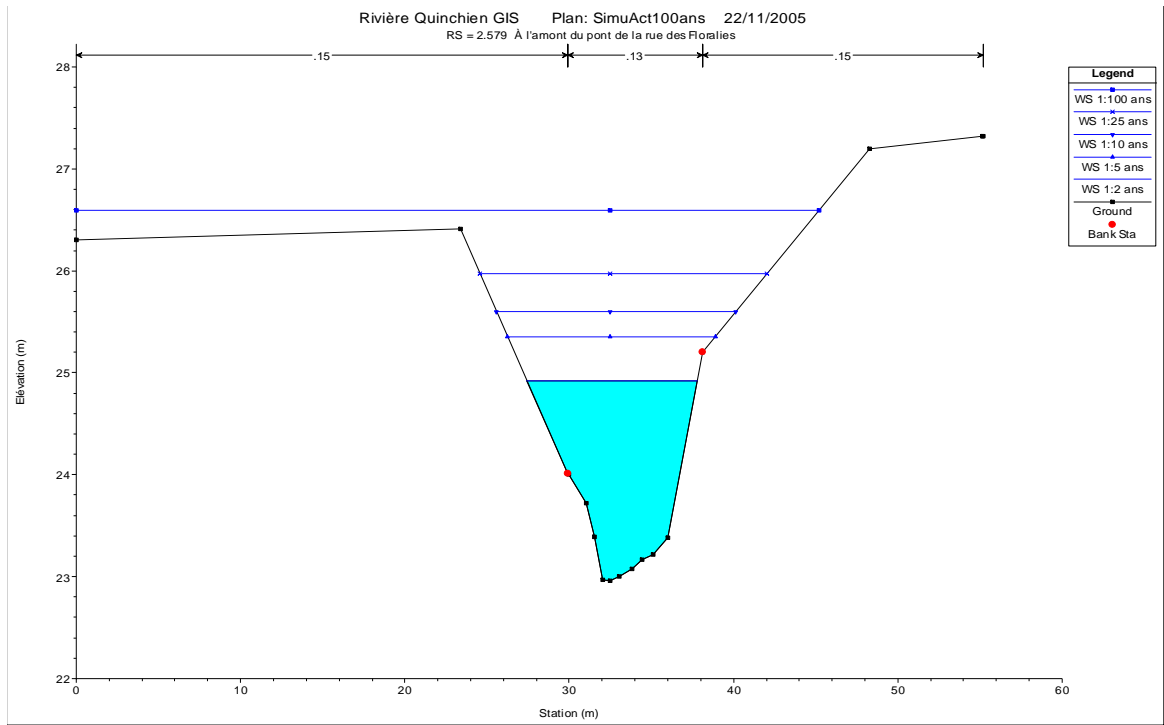
C-9a. Niveaux calculés avec le bassin actuel au ch 2+579
