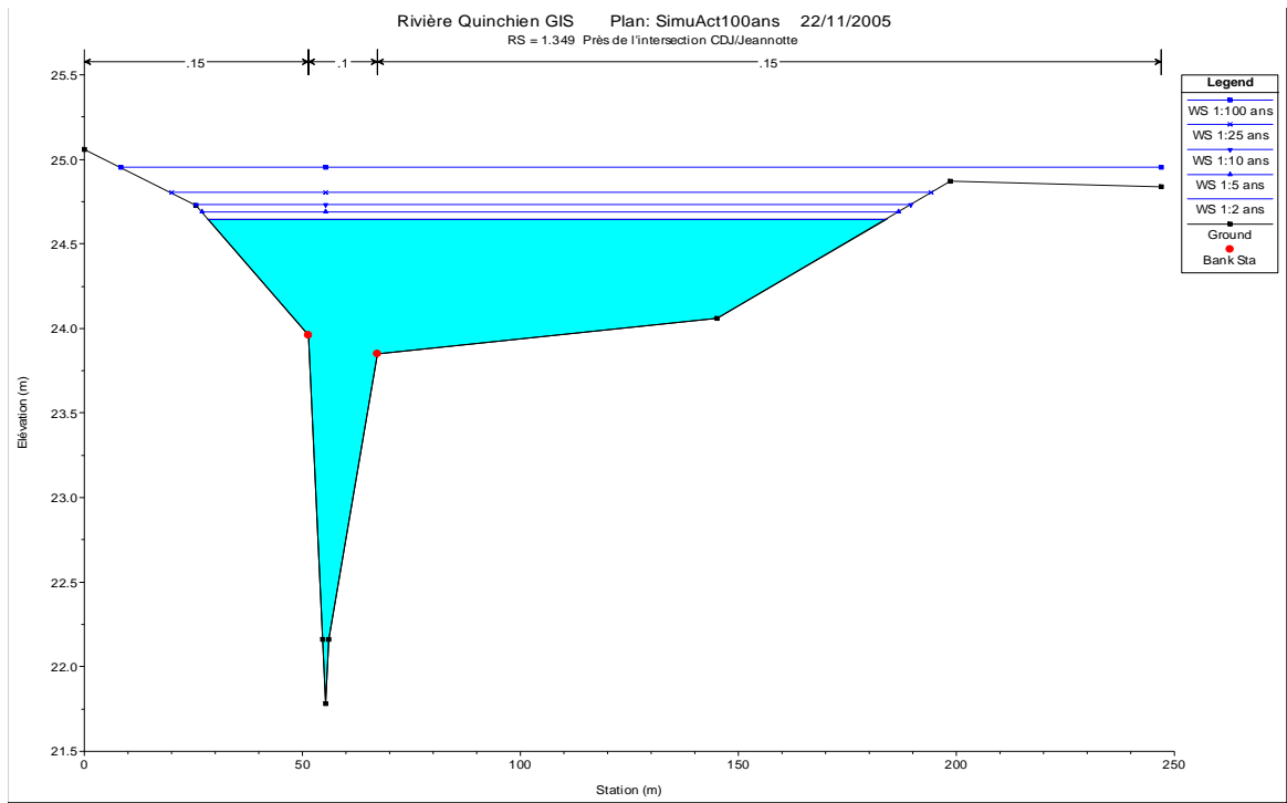
C-4a. Niveaux calculés avec le bassin actuel au ch 1+349
