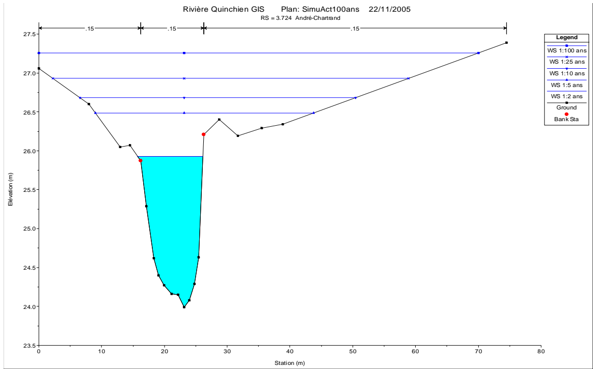
C-10a. Niveaux calculés avec le bassin actuel au ch 3+724
