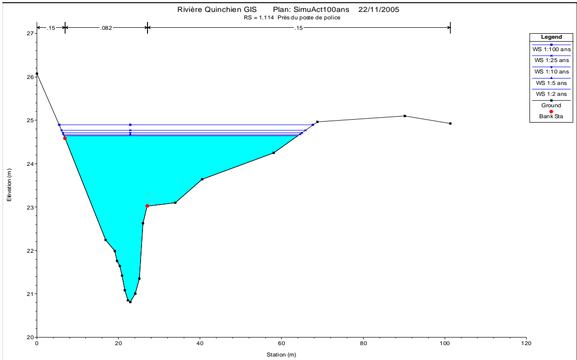
C-2a. Niveaux calculés avec le bassin actuel au ch 1+114
