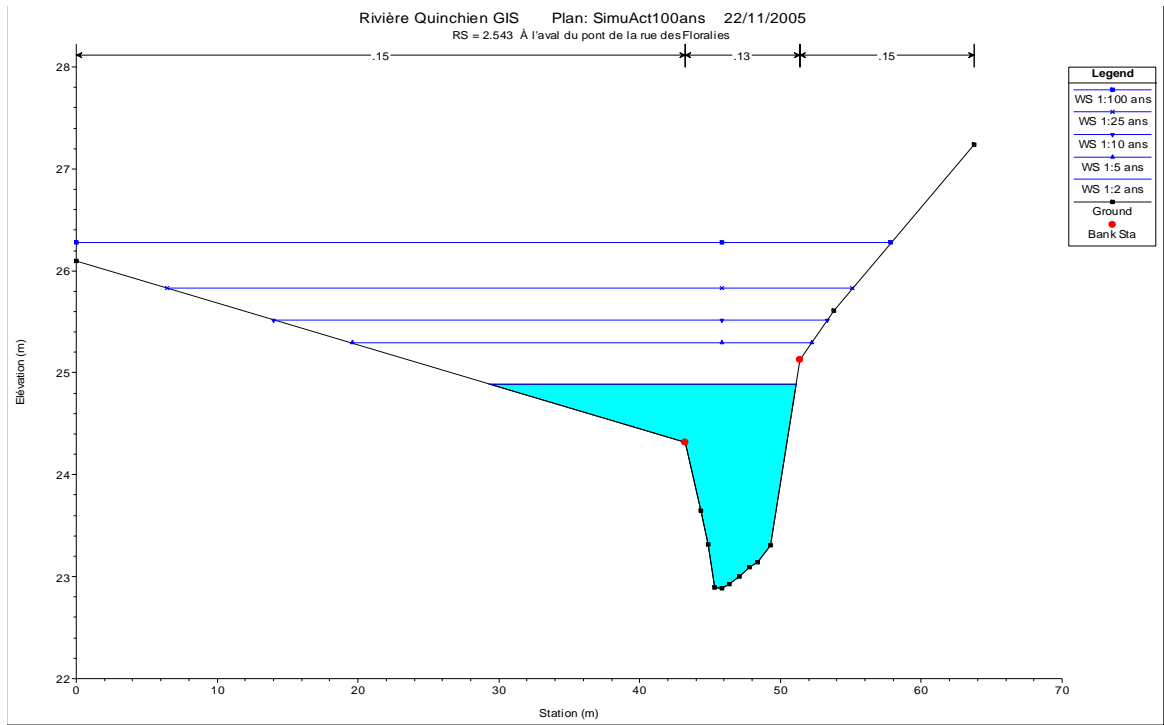
C-8a. Niveaux calculés avec le bassin actuel au ch 2+543
