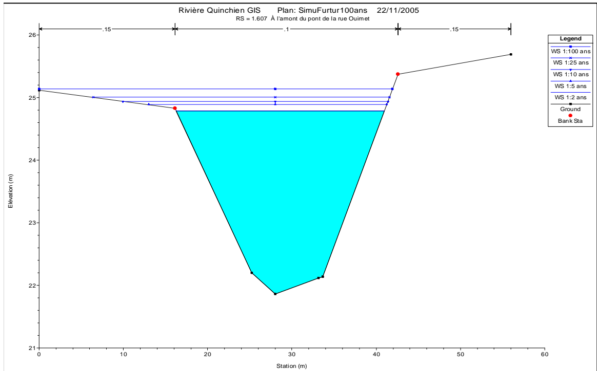
C-6b. Niveaux calculés avec le bassin futur au ch 1+607
