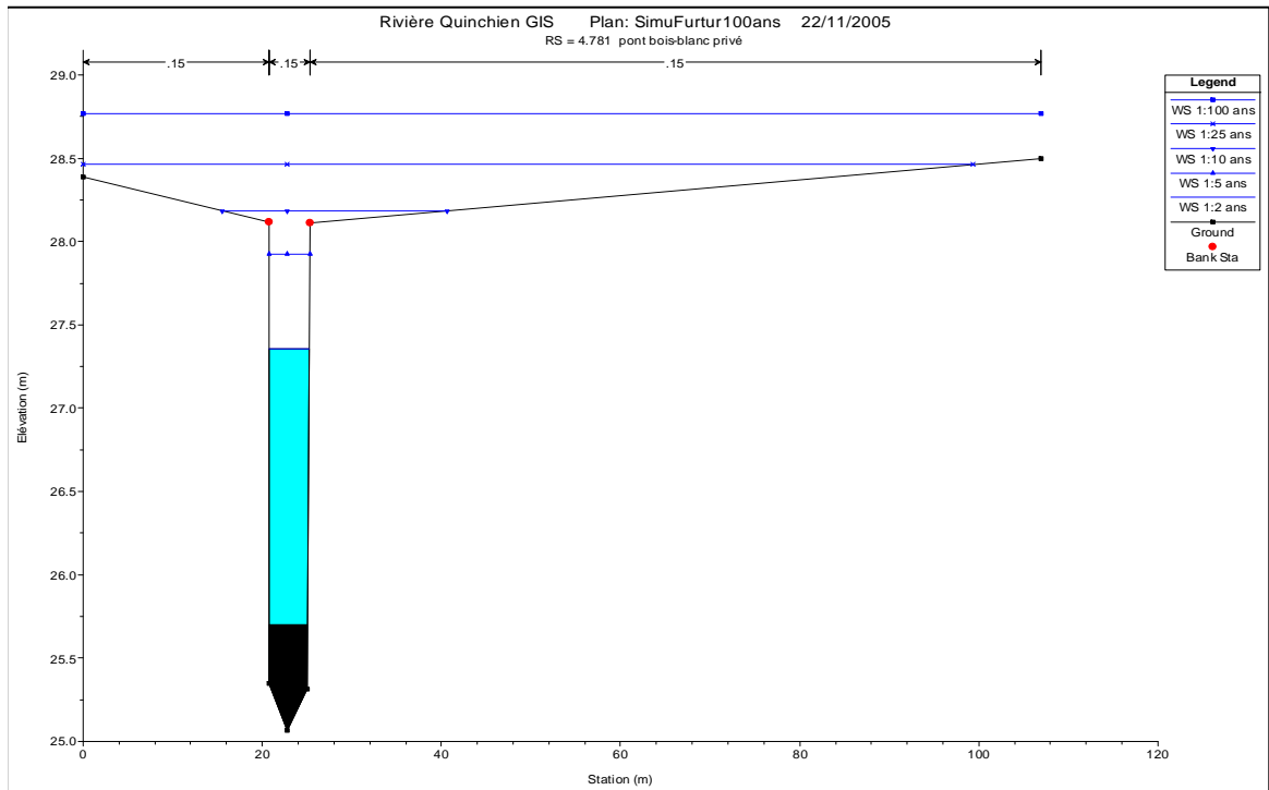
C-11b. Niveaux calculés avec le bassin futur au ch 4+781
