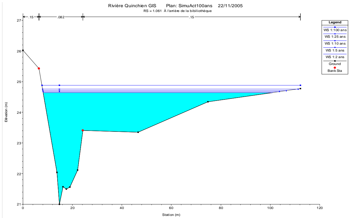
C-1a. Niveaux calculés avec le bassin actuel au ch 1+061
