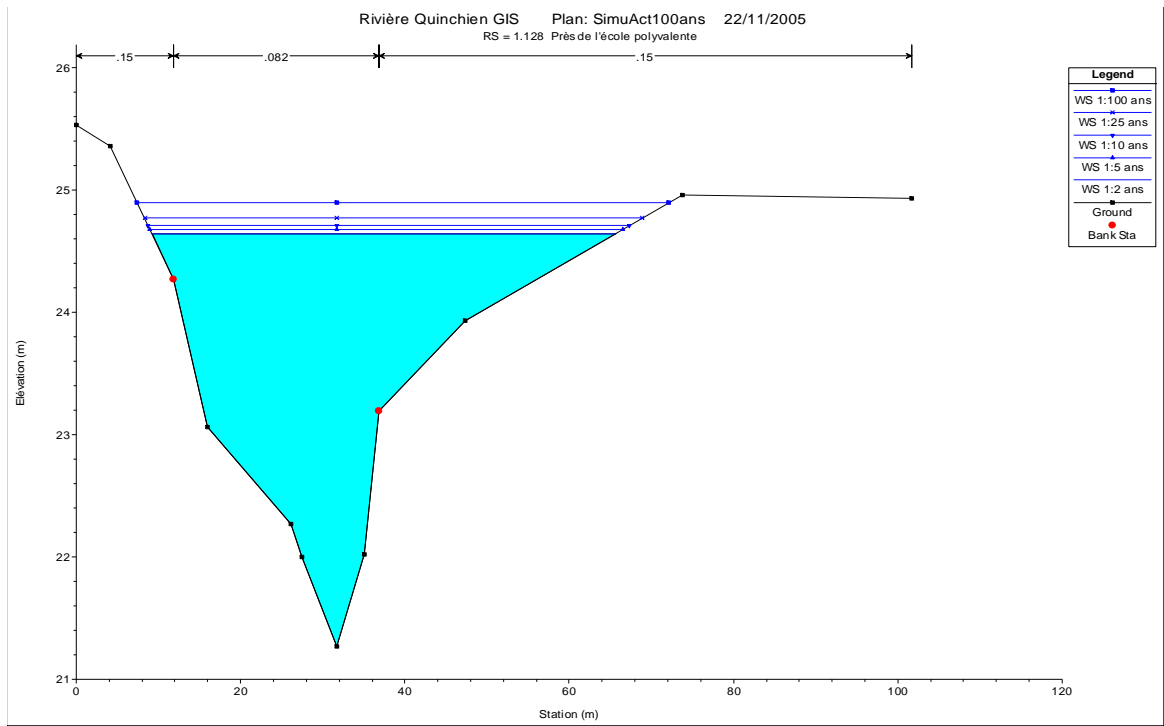
C-3a. Niveaux calculés avec le bassin actuel au ch 1+128
