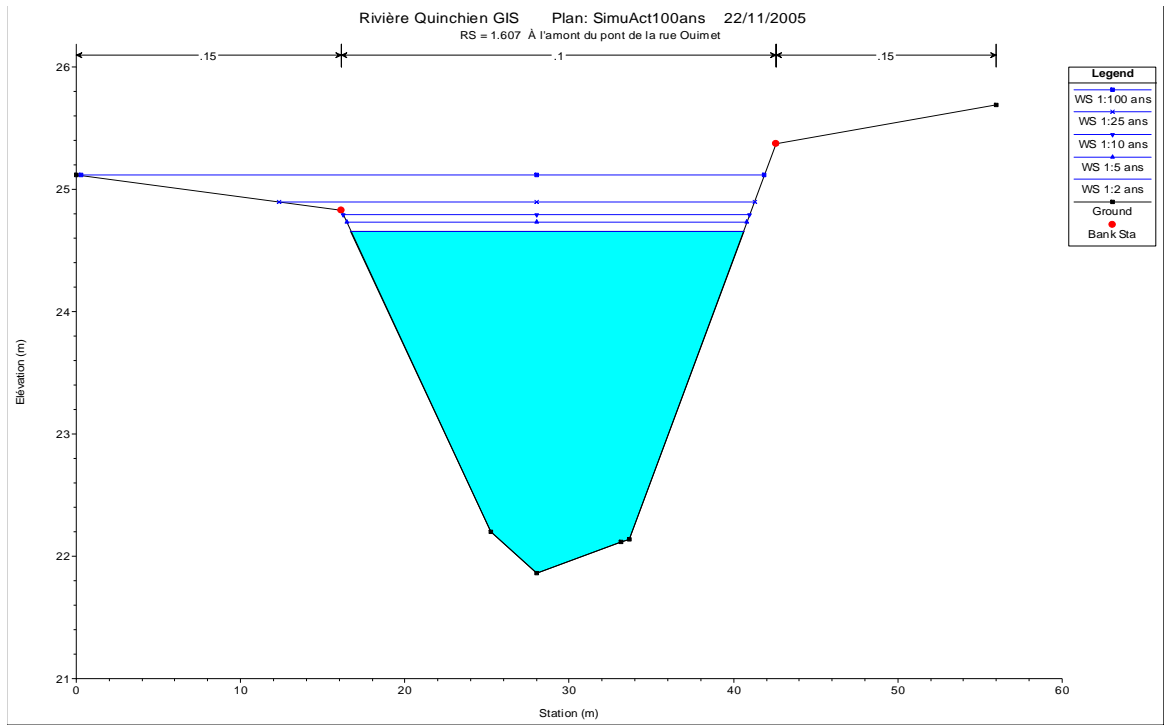
C-6a. Niveaux calculés avec le bassin actuel au ch 1+607
