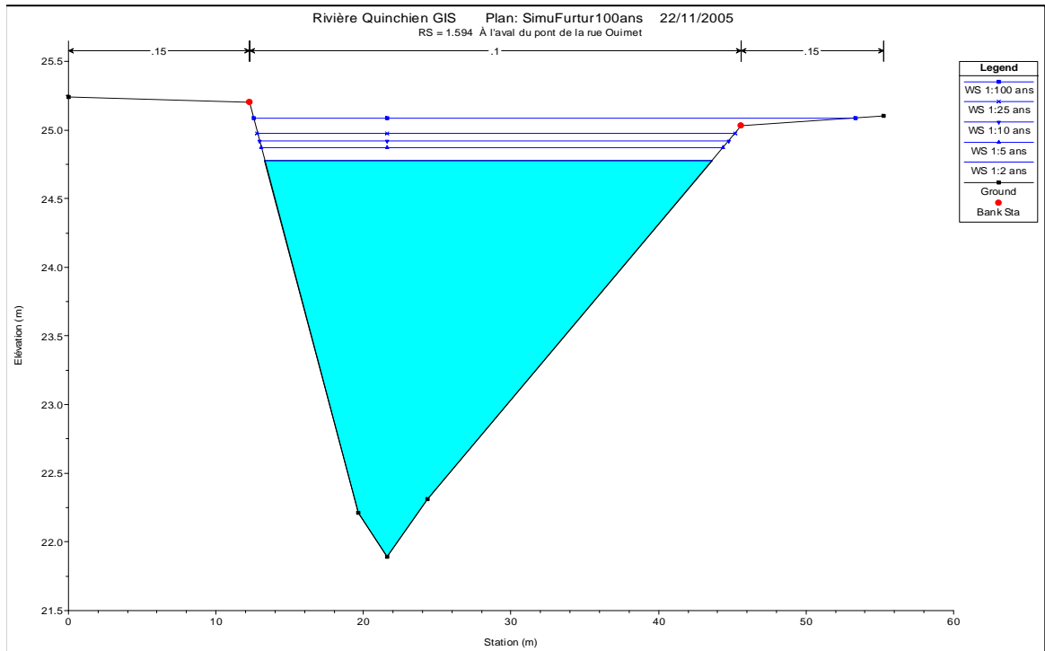
C-5b. Niveaux calculés avec le bassin futur au ch 1+594
