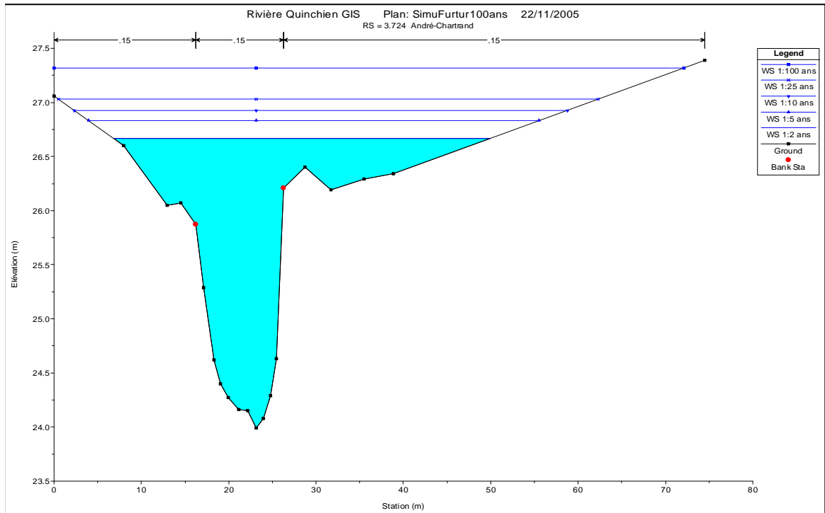
C-10b. Niveaux calculés avec le bassin futur au ch 3+724
