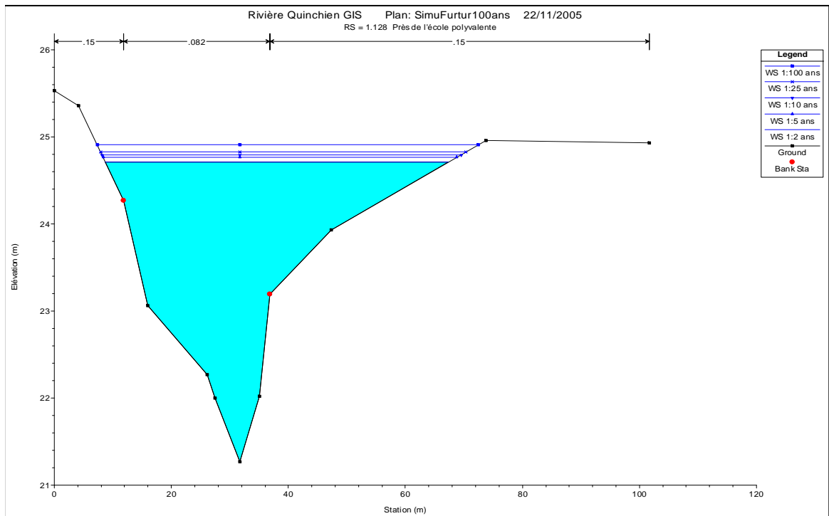
C-3b. Niveaux calculés avec le bassin futur au ch 1+128
