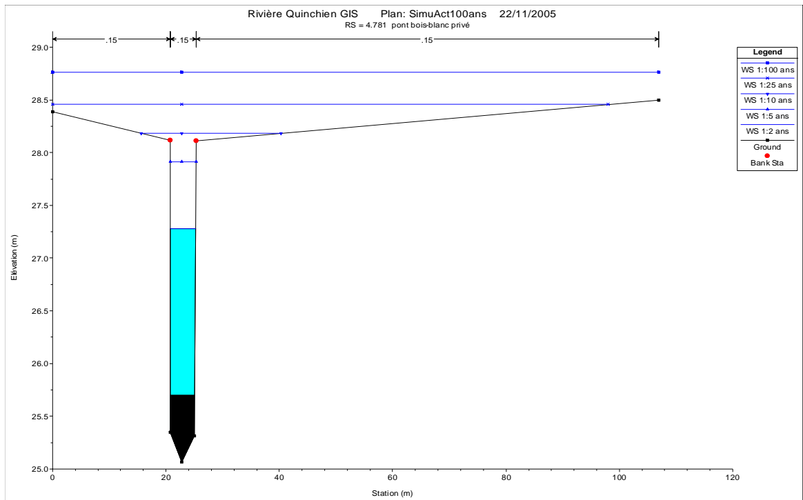
C-11a. Niveaux calculés avec le bassin actuel au ch 4+781
