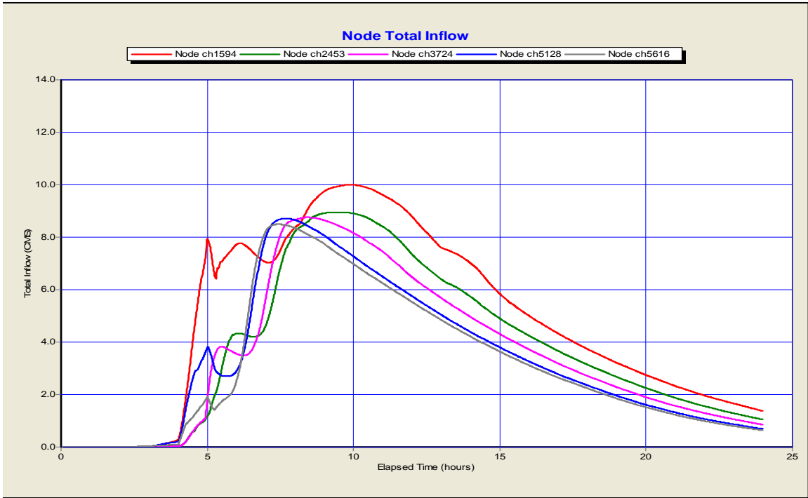
Figure B-3 Hydrographes de la rivière Quinchien en condition actuelle et à la pluie de 1:10 ans
