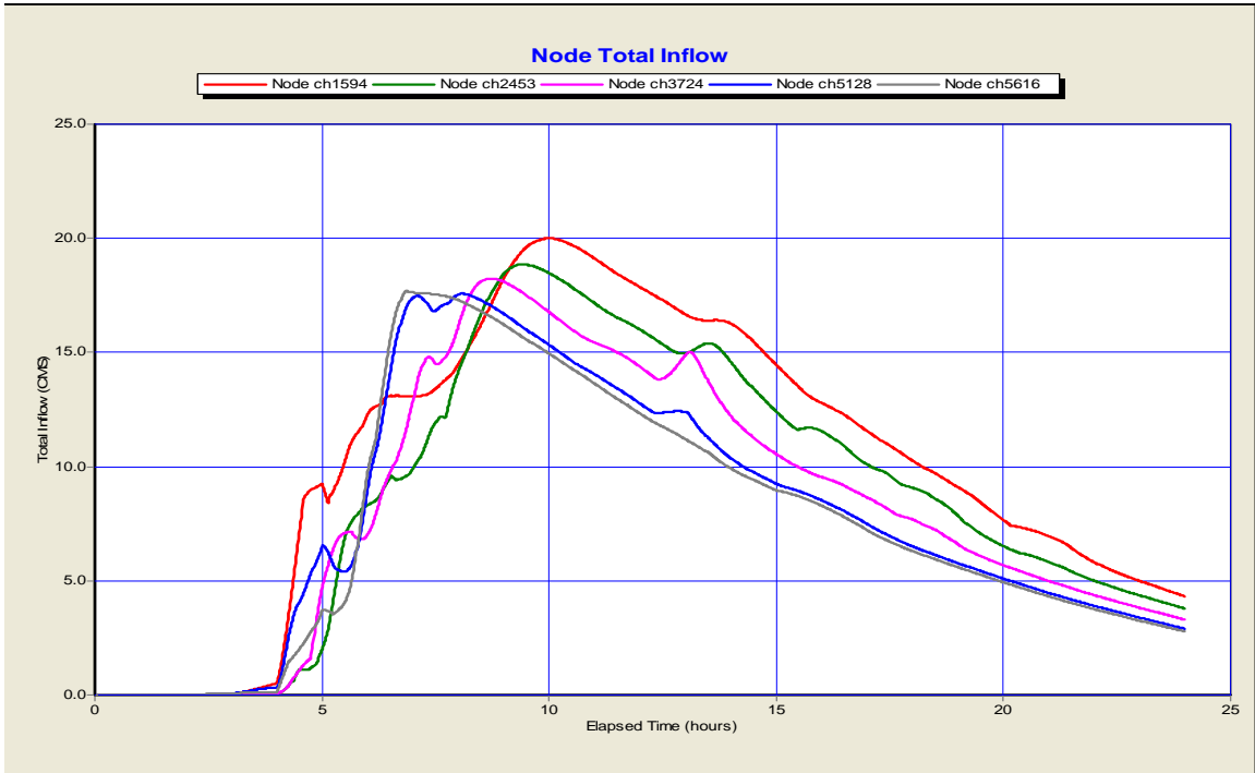
Figure B-1 Hydrographes de la rivière Quinchien en condition actuelle et à la pluie de 1:100ans
