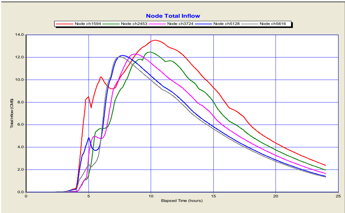
Figure B-2 Hydrographes de la rivière Quinchien en condition actuelle et à la pluie de 1:25 ans
