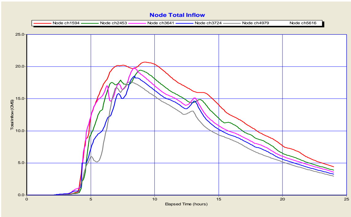
Figure B-5 Hydrographes de la rivière Quinchien en condition futur et à la pluie de 1:100 ans
