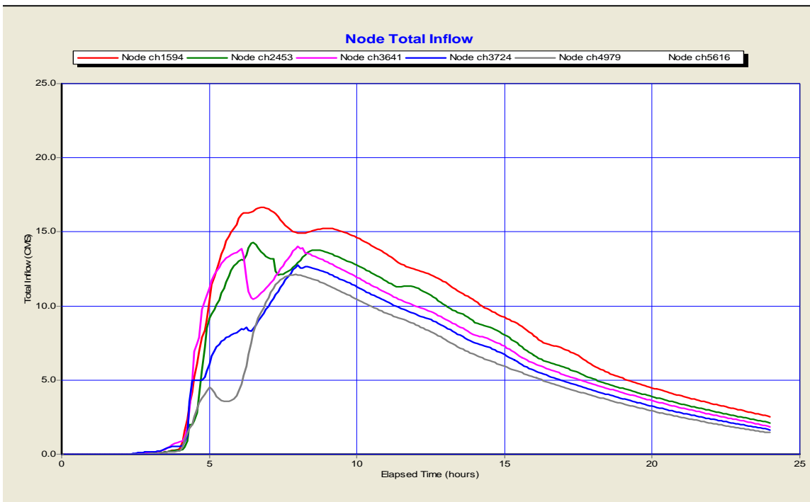
Figure B-6 Hydrographes de la rivière Quinchien en condition futur et à la pluie de 1:25 ans
