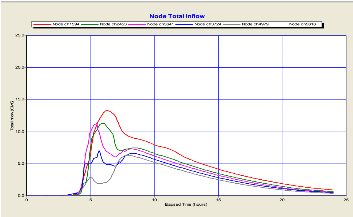
Figure B-8 Hydrographes de la rivière Quinchien en condition futur et à la pluie de 1:5 ans
