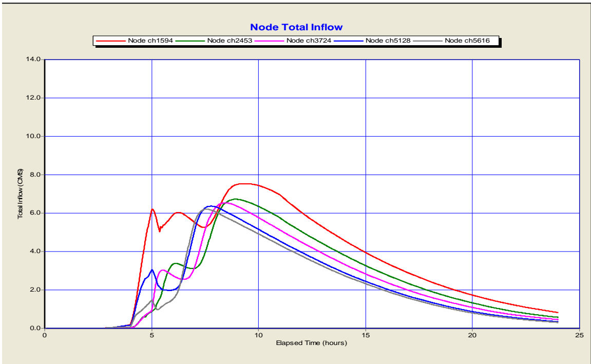
Figure B-4 Hydrographes de la rivière Quinchien en condition actuelle et à la pluie de 1:5 ans
