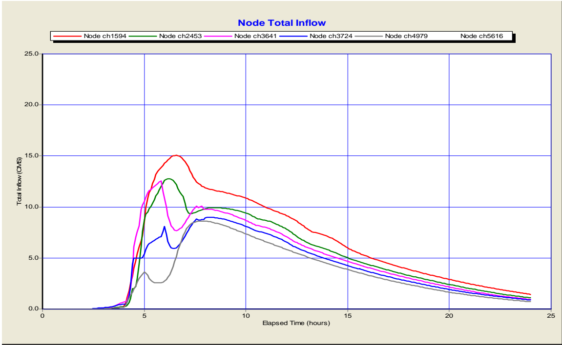
Figure B-7 Hydrographes de la rivière Quinchien en condition futur et à la pluie de 1:10 ans
