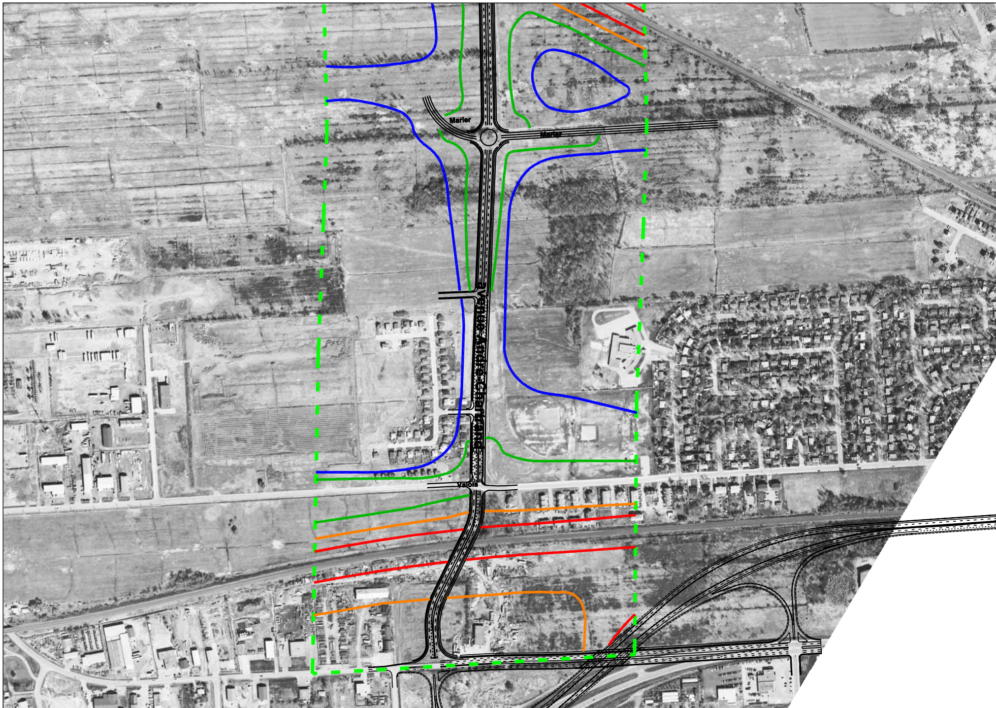
Groupe Conseil Génivar Figure 17 : Climat sonore projeté scénario 2 avec mesures correctives (André-Chartrand 2)
