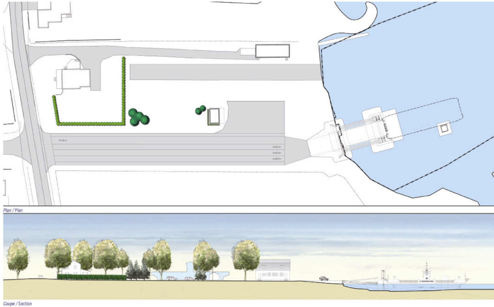
Figure 4 – Schéma des installations projetées à Hudson.
