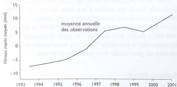
Figure 0.1. Élévation du niveau moyen de l'océan entre 1993 et 2001 (environ 2 centimètres) mesurée par le satellite Topex-Poseidon. Cette
