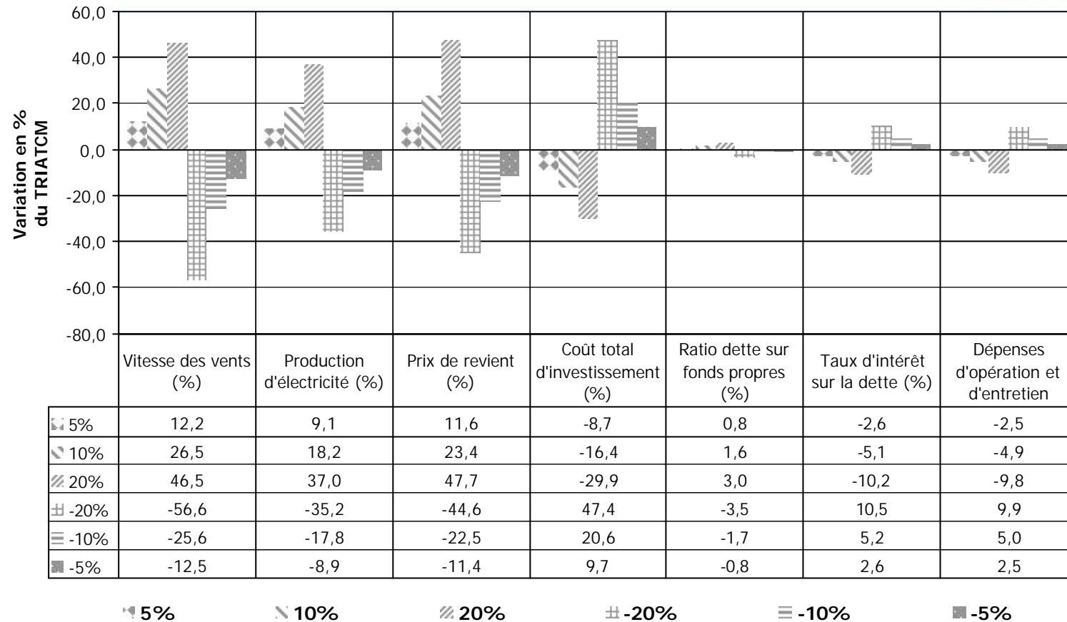
Figure 4.2 : Résultats de la sensibilité du TRIATCM après taxes sur le capital et municipales à la variation de sept paramètres
