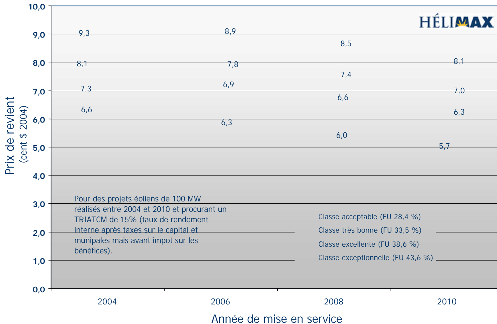
Figure 4.1 : Prix de revient de l'énergie éolienne au Québec selon l'évolution technologique pour 4 classes de gisement
