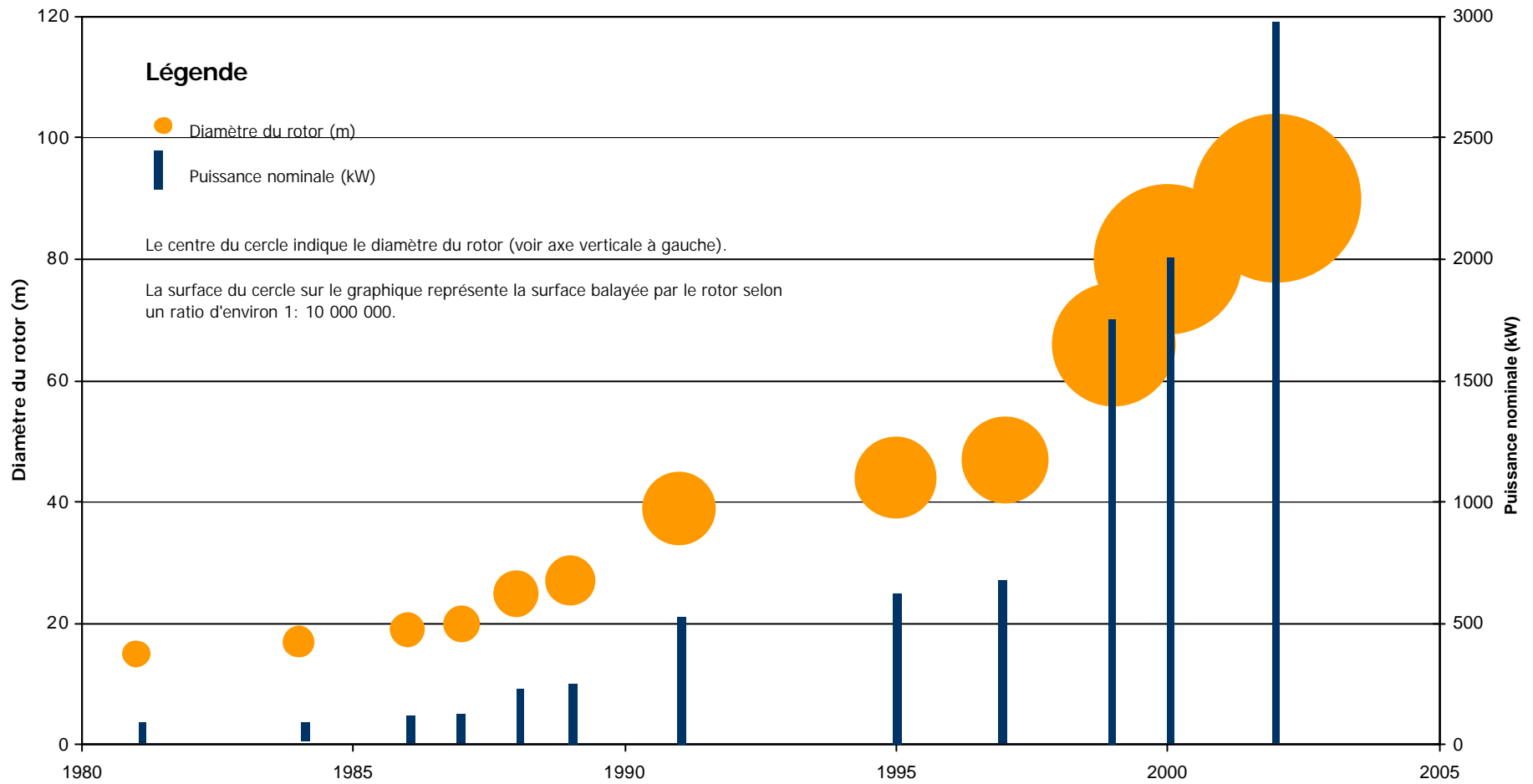
Figure 2.3 : Évolution de la taille des éoliennes sur la période de 1980 à 2005
