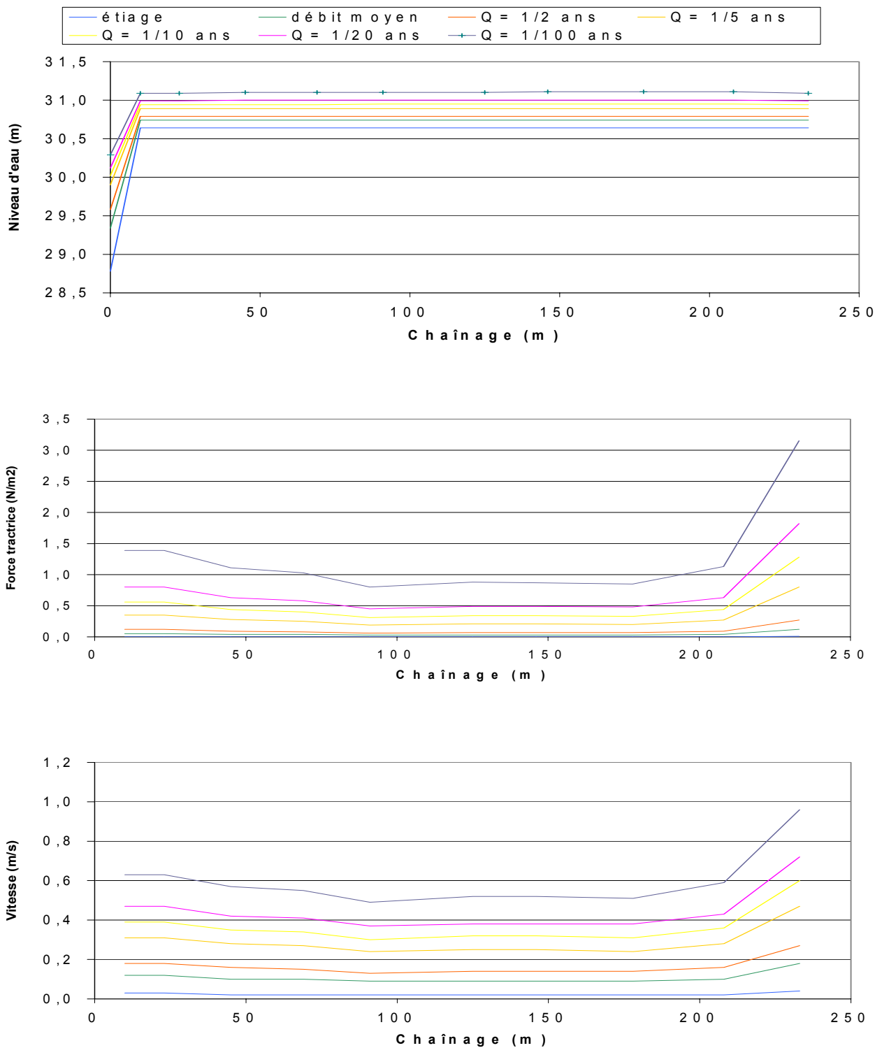
Figure 3-6 : Caractéristiques hydrauliques de la rivière Saint-Louis en amont de la digue Howard-Smith, en condition estivale - Niveau, force tractrice et vitesse du courant
