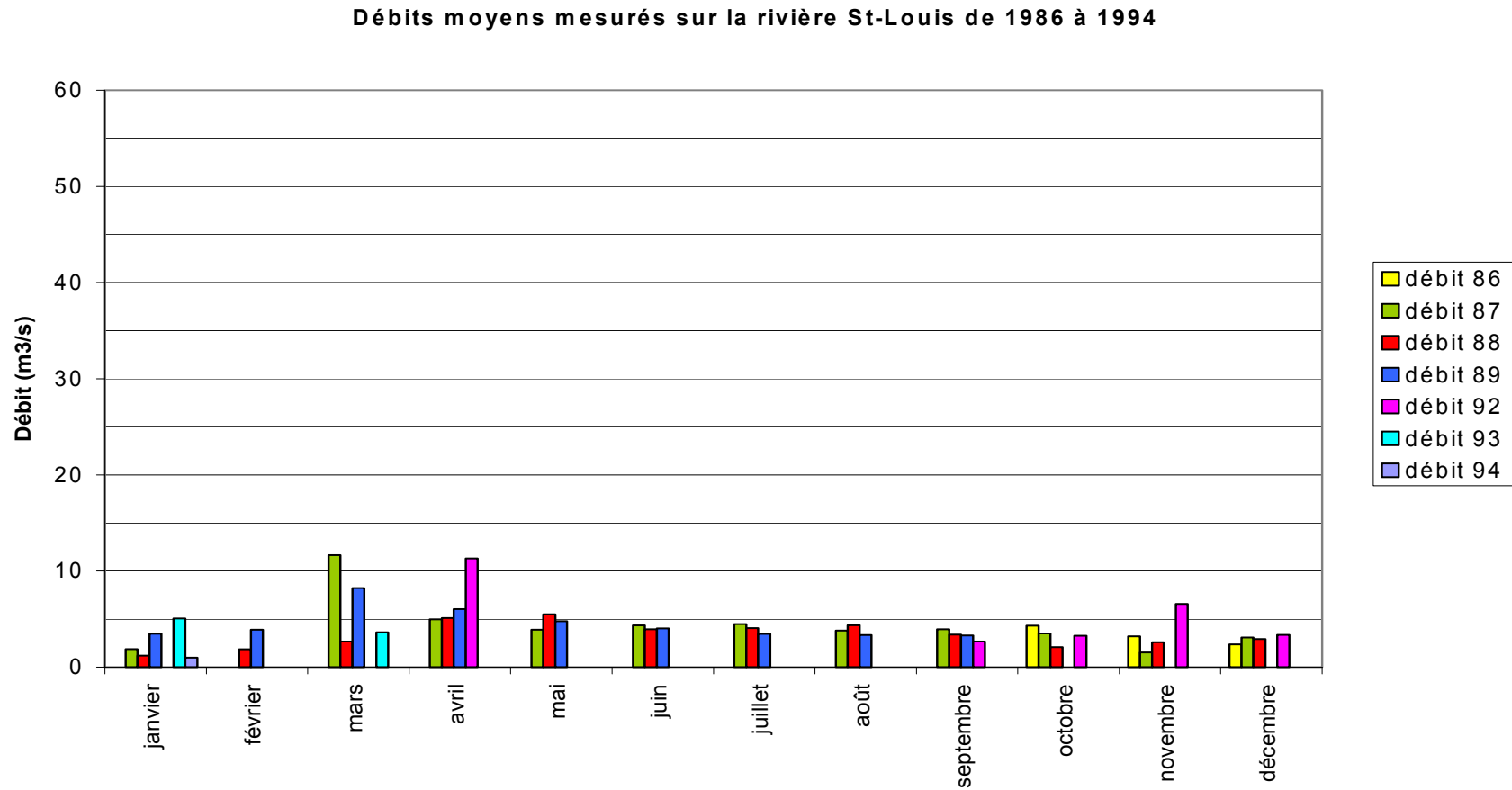
Figure 3-4 : Débits moyens (1986-1994) de la rivière Saint-Louis
