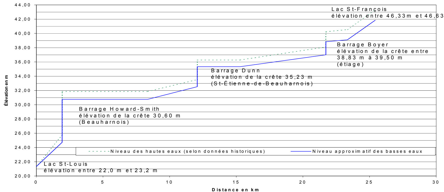
Figure 3-3 : Profil du cours d'eau de la rivière Saint-Louis
