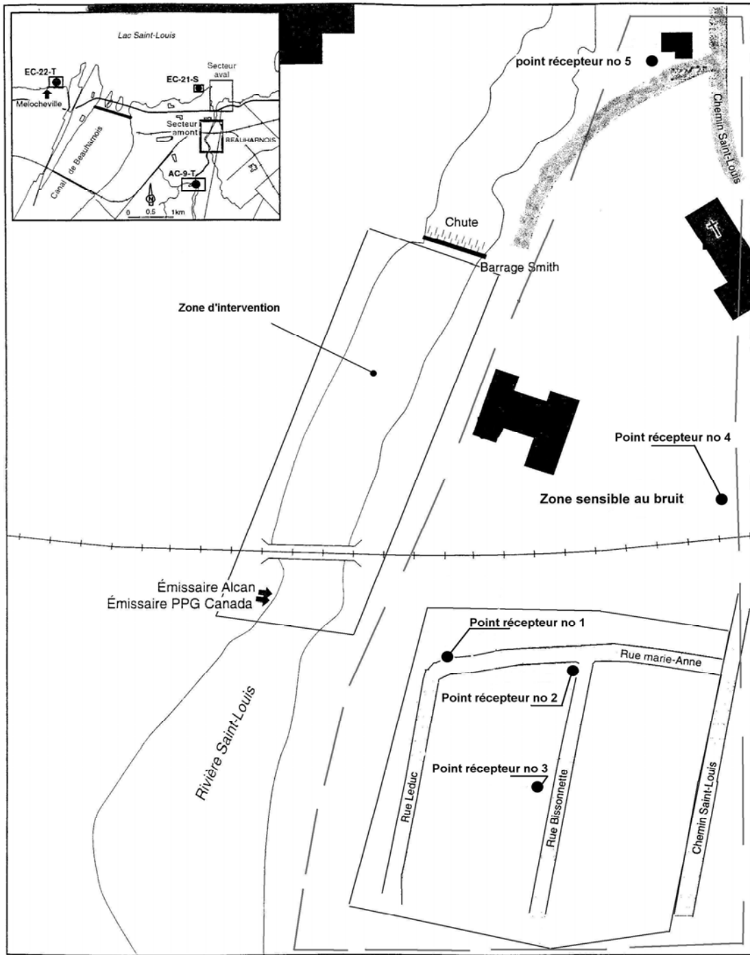
Figure 3-13 : Localisation des points de mesures des niveaux sonores dans les zones résidentielles
