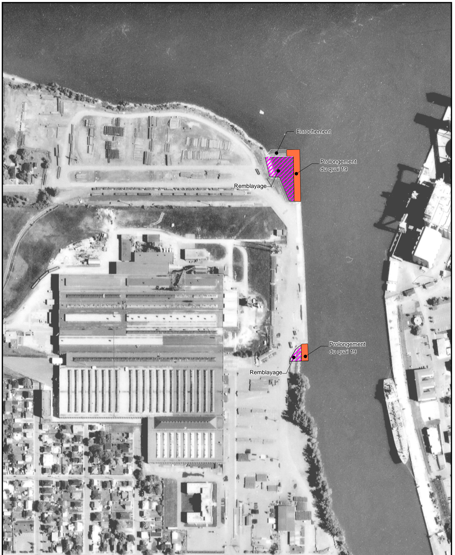
Figure 3.3 Variante C ( 75 m vers le nord et 25 m au sud )
