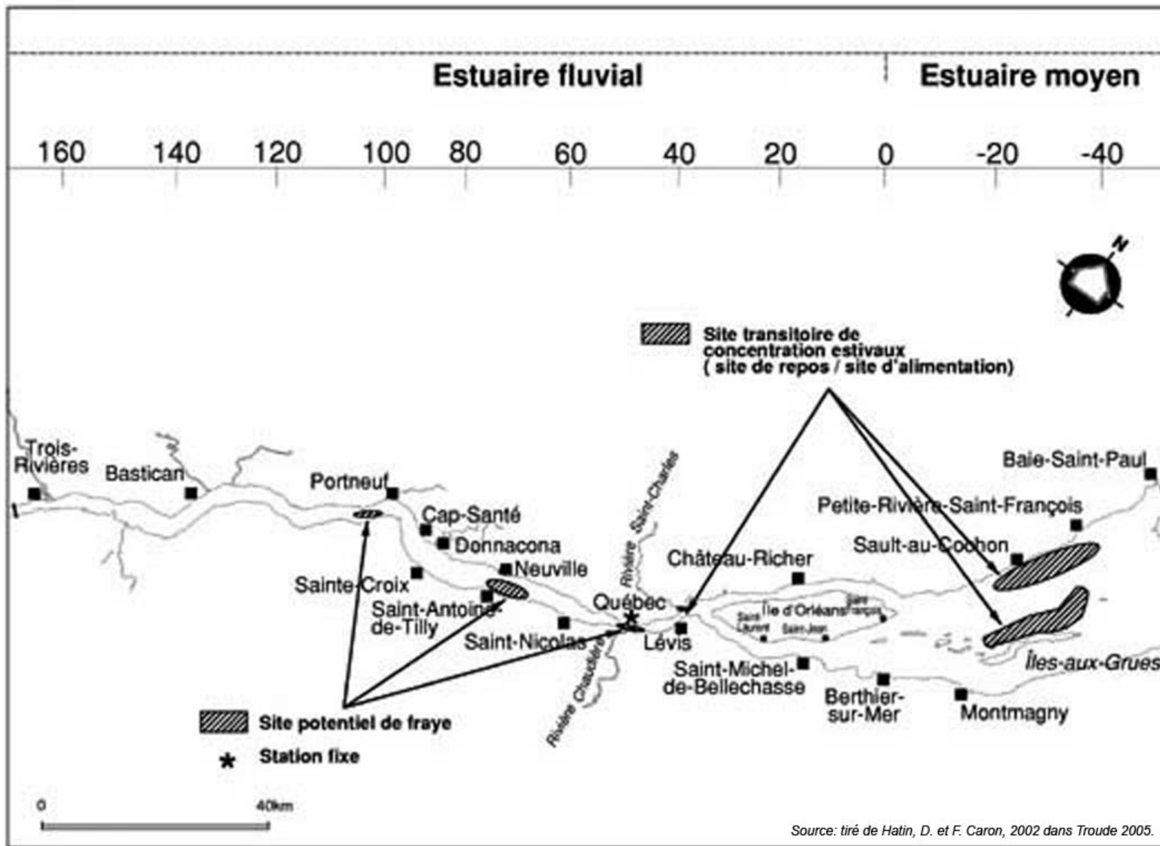
FIGURE 2.15 Identification des zones d'alimentation estivales (en aval) et des sites potentiels de fraye (en amont) pour l'esturgeon noir
