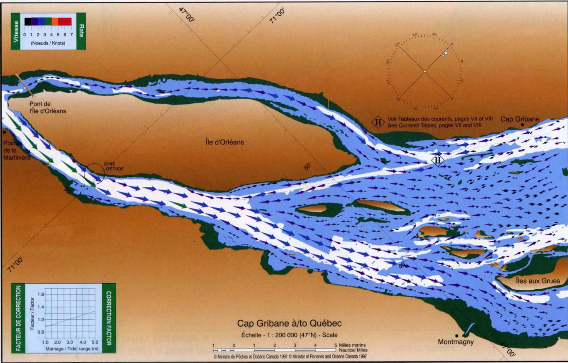
FIGURE 2.4 Courantométrie
