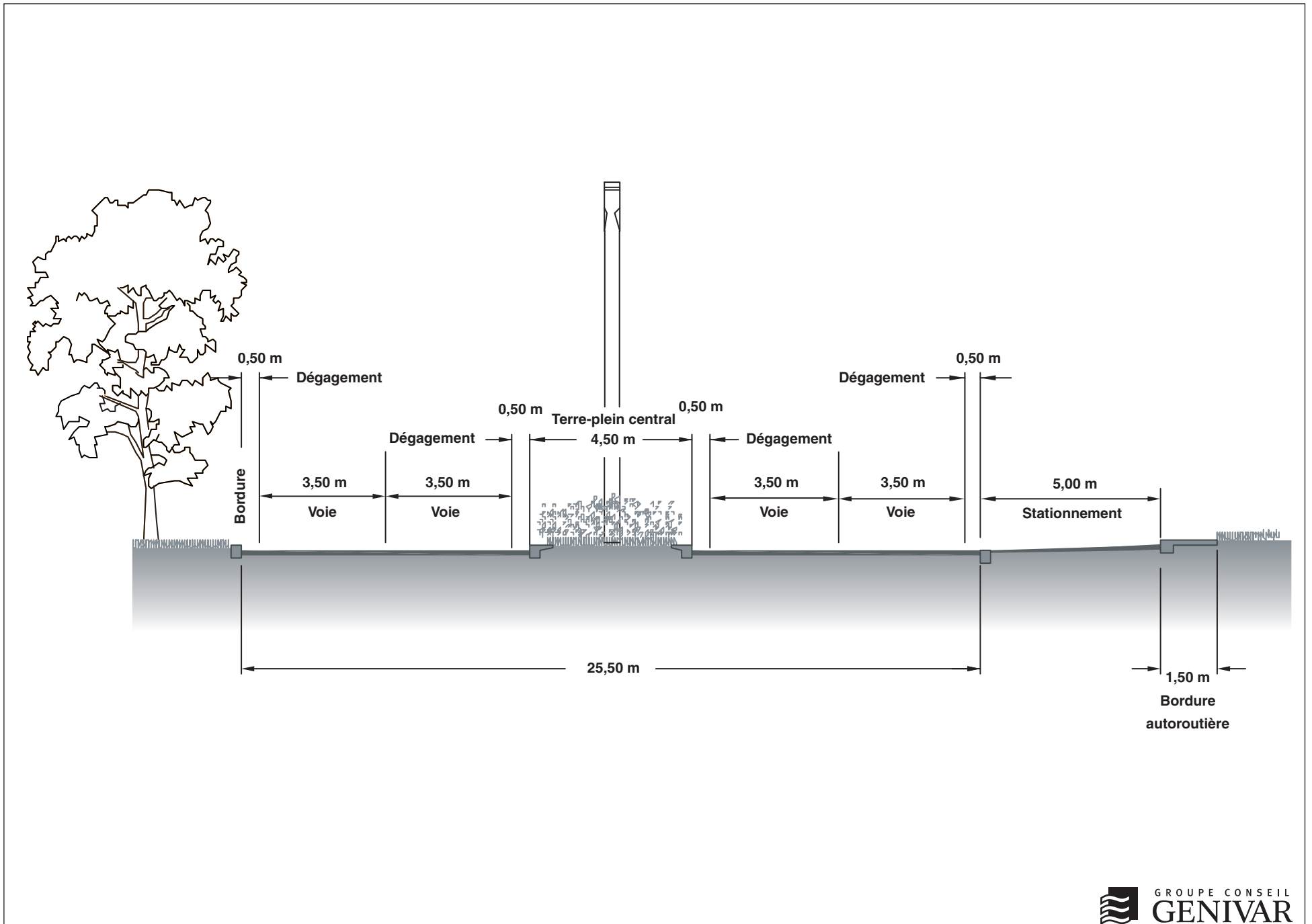
Figure 4.3 Profil en travers proposé du boulevard Champlain.
