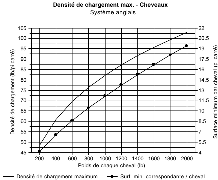
Figure 6 Espace minimum à allouer pour les cervidés durant le transport selon le poids corporel individuel (syst. métrique). L'axe de gauche donne le poids maximum par unité de surface du plancher, et l'axe de droite donne la surface minimum correspondante par animal. Les cervidés devraient disposer d'assez d'espace pour pouvoir tous se coucher, quelle que soit la durée du trajet.
