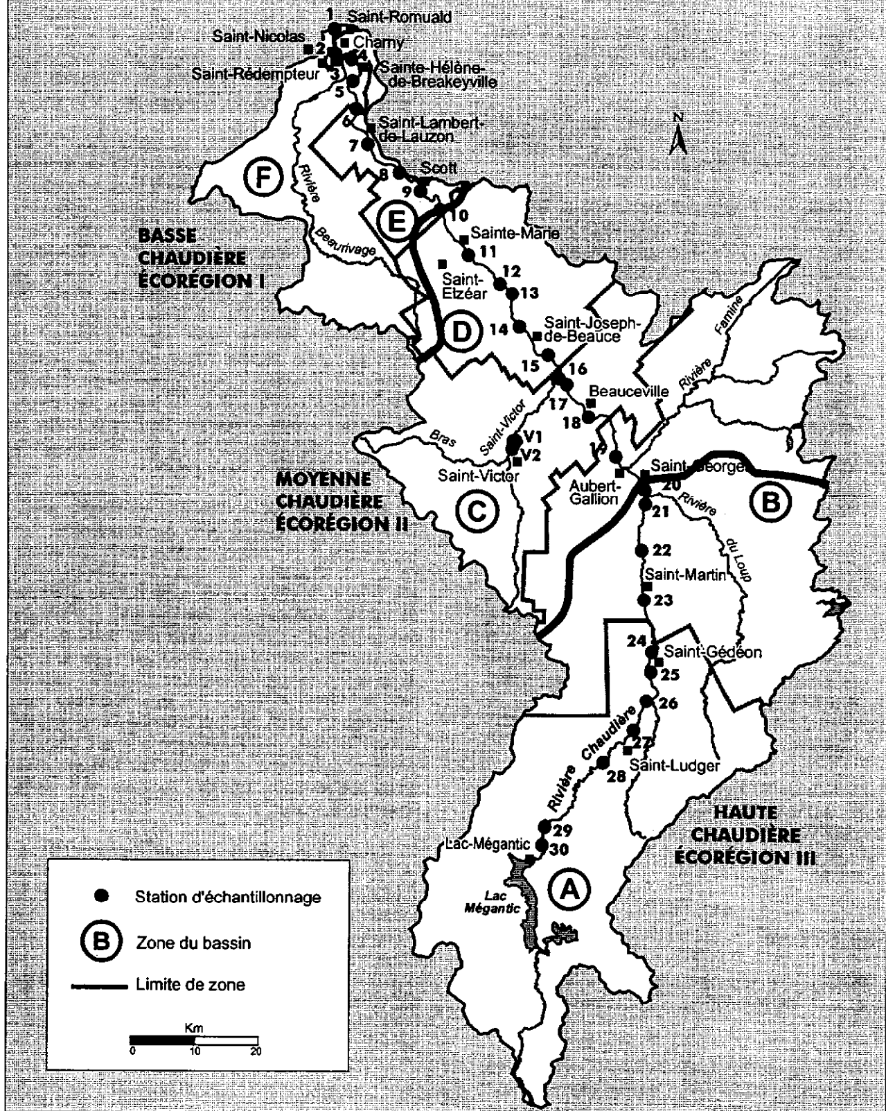
Figure 1 Localisation des écorégions du bassin versant de la rivière Chaudière et des stations d'échantillonnage de la qualité de l'eau et des communautés ichthyologiques et benthiques
