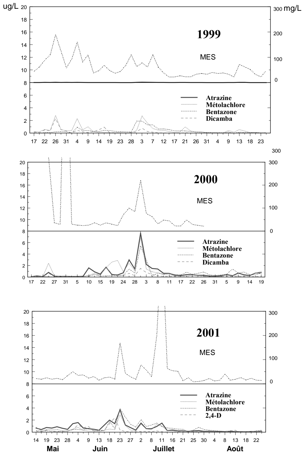
Figure 7 Comparaison des concentrations de MES et d'herbicides dans la rivière des Hurons
