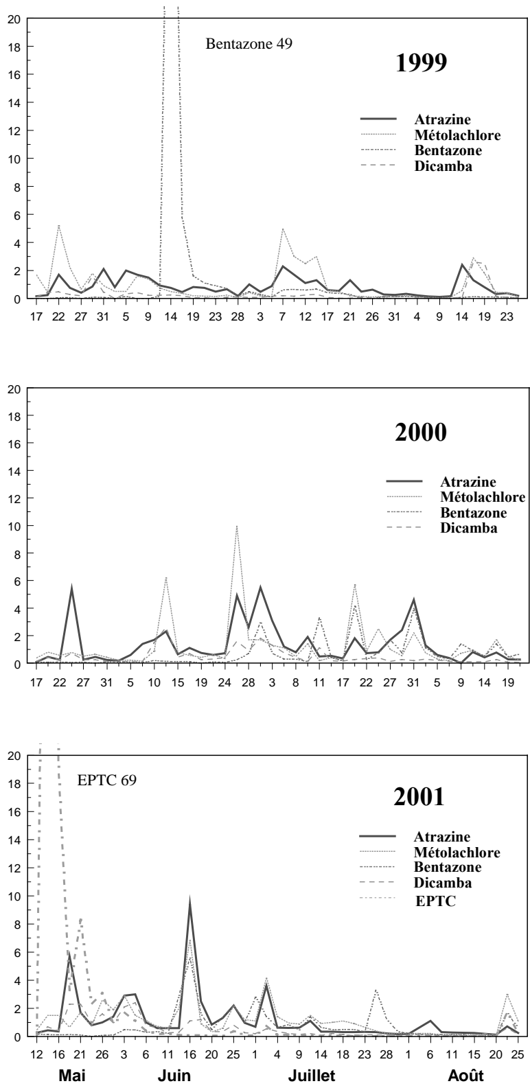
Figure 4 Concentrations de quelques herbicides décelés dans la rivière Saint-Régis (µg/L)
