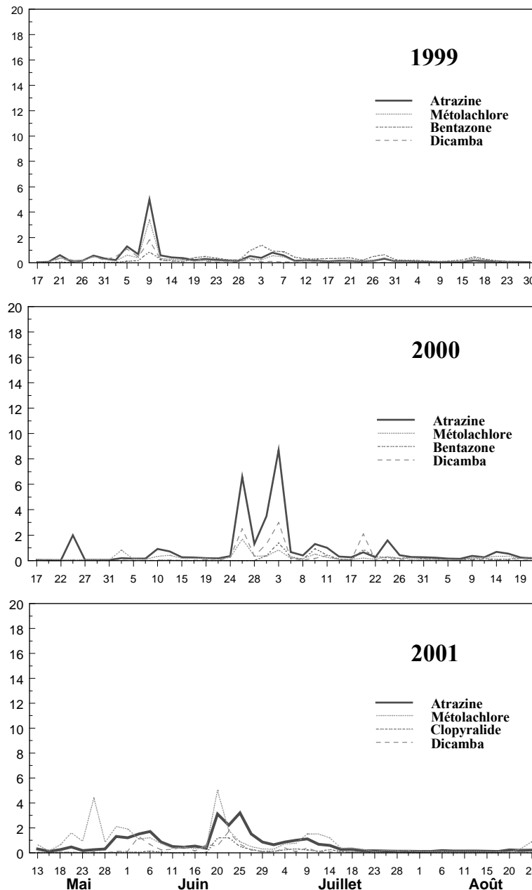
Figure 5 Concentrations de quelques herbicides décelés dans la rivière Saint-Zéphirin (µg/L)
