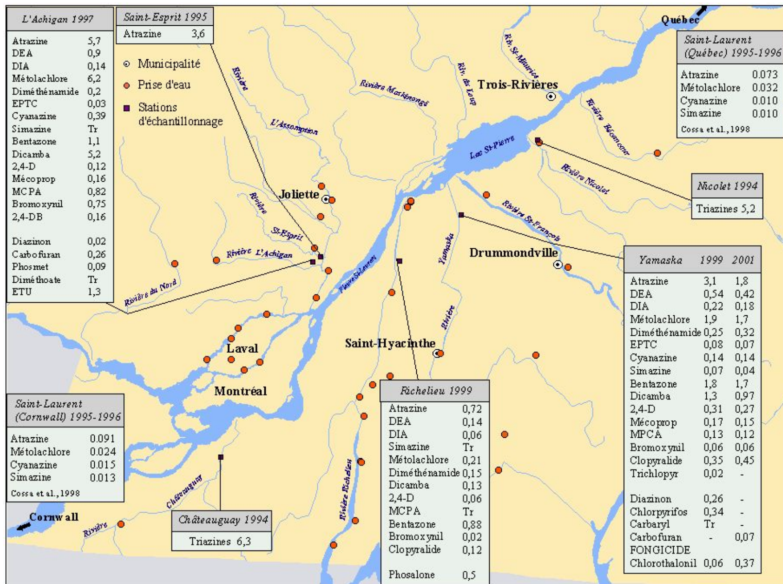
Figure 9 Concentrations maximales de pesticides dans l'eau brute de quelques cours d'eau servant de source d'alimentation en eau potable
