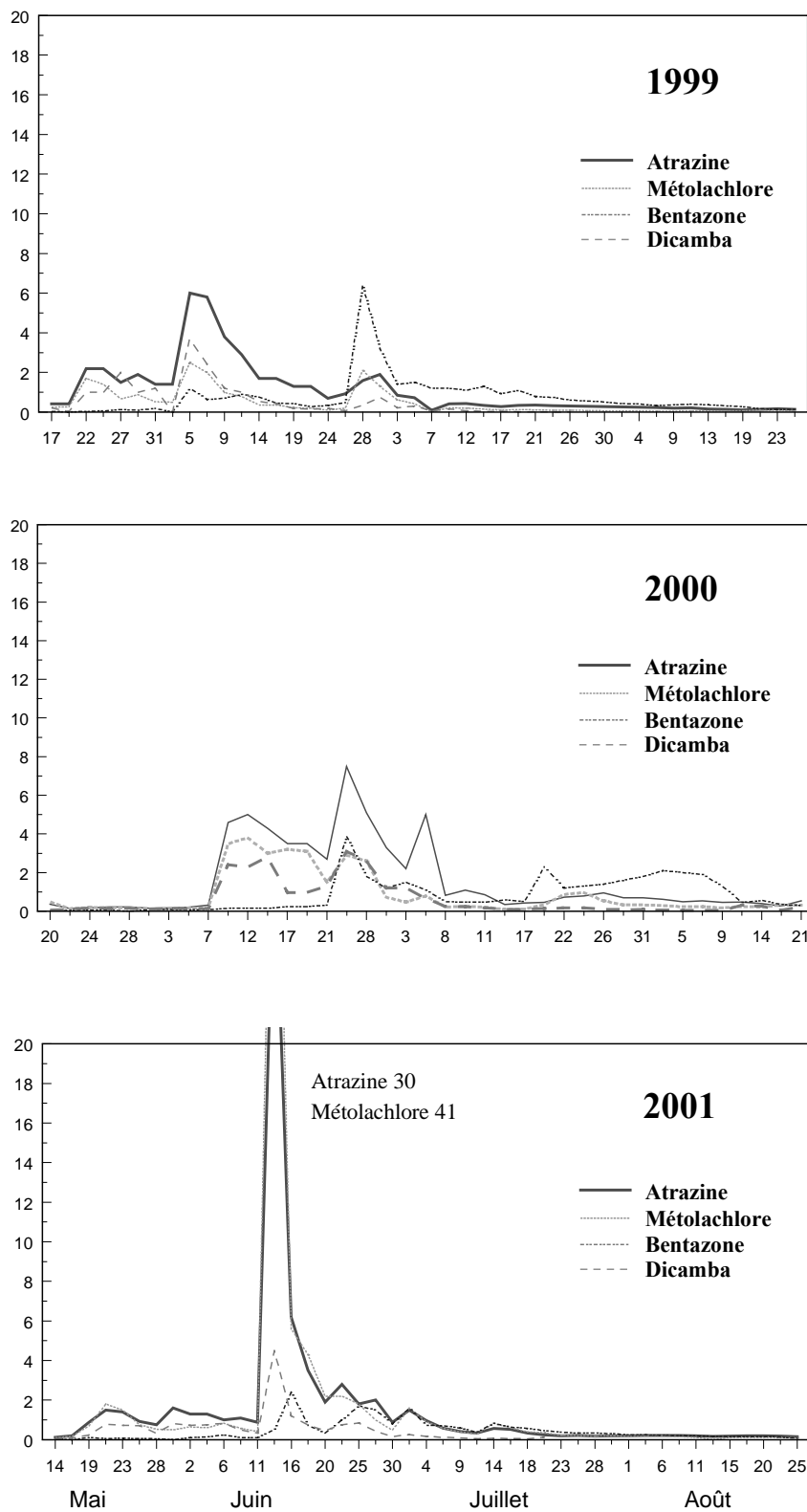
Figure 2 Concentrations de quelques herbicides décelés dans la rivière Chibouet ( \mu\text{g/L} )
