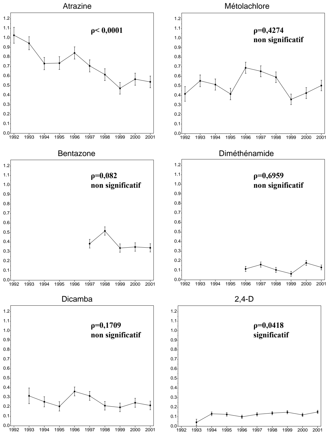
Figure 6 Tendances temporelles des concentrations moyennes* pour quelques herbicides
