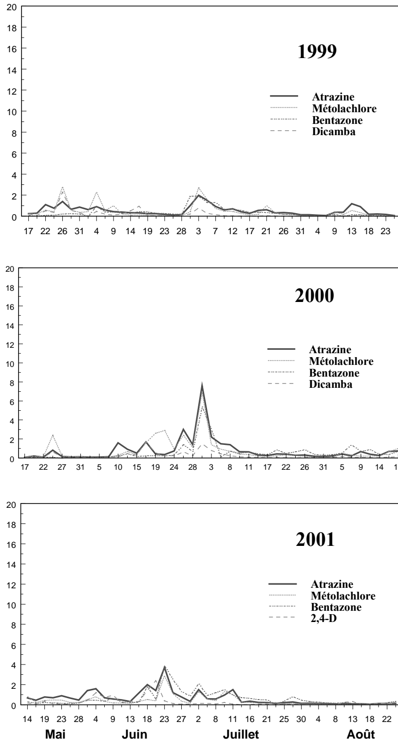
Figure 3 Concentrations de quelques herbicides dans la rivière des Hurons (µg/L)
