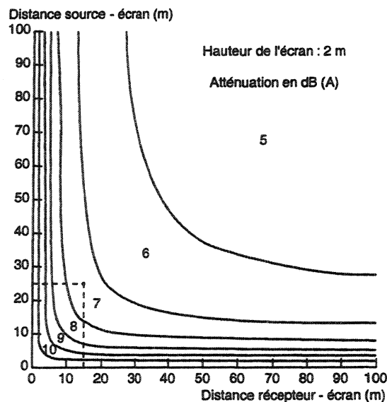
Fig. 3 - Atténuation due à la présence d'un écran.
