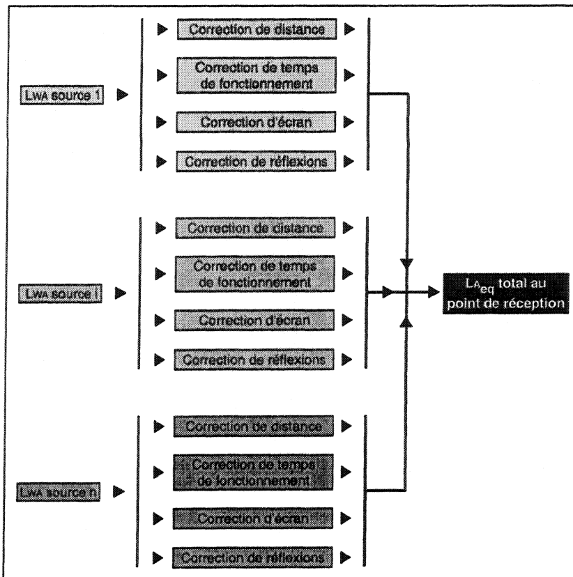
Fig. 2 - Principe général de la méthode du Laboratoire régional des Ponts et Chaussées de Blois.
