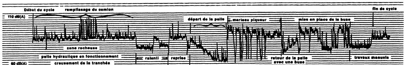
Fig. 1 - Chantier d'assainissement en milieu urbain.
