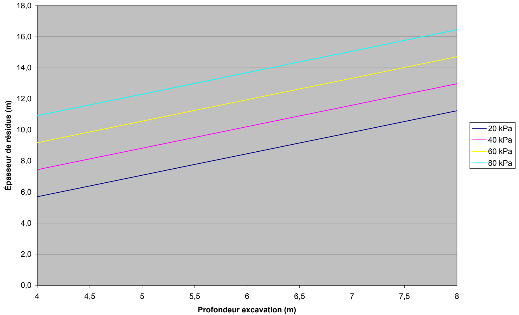
Fig 9-2 : Relation profondeur d'excavation vs épaisseur de résidus
