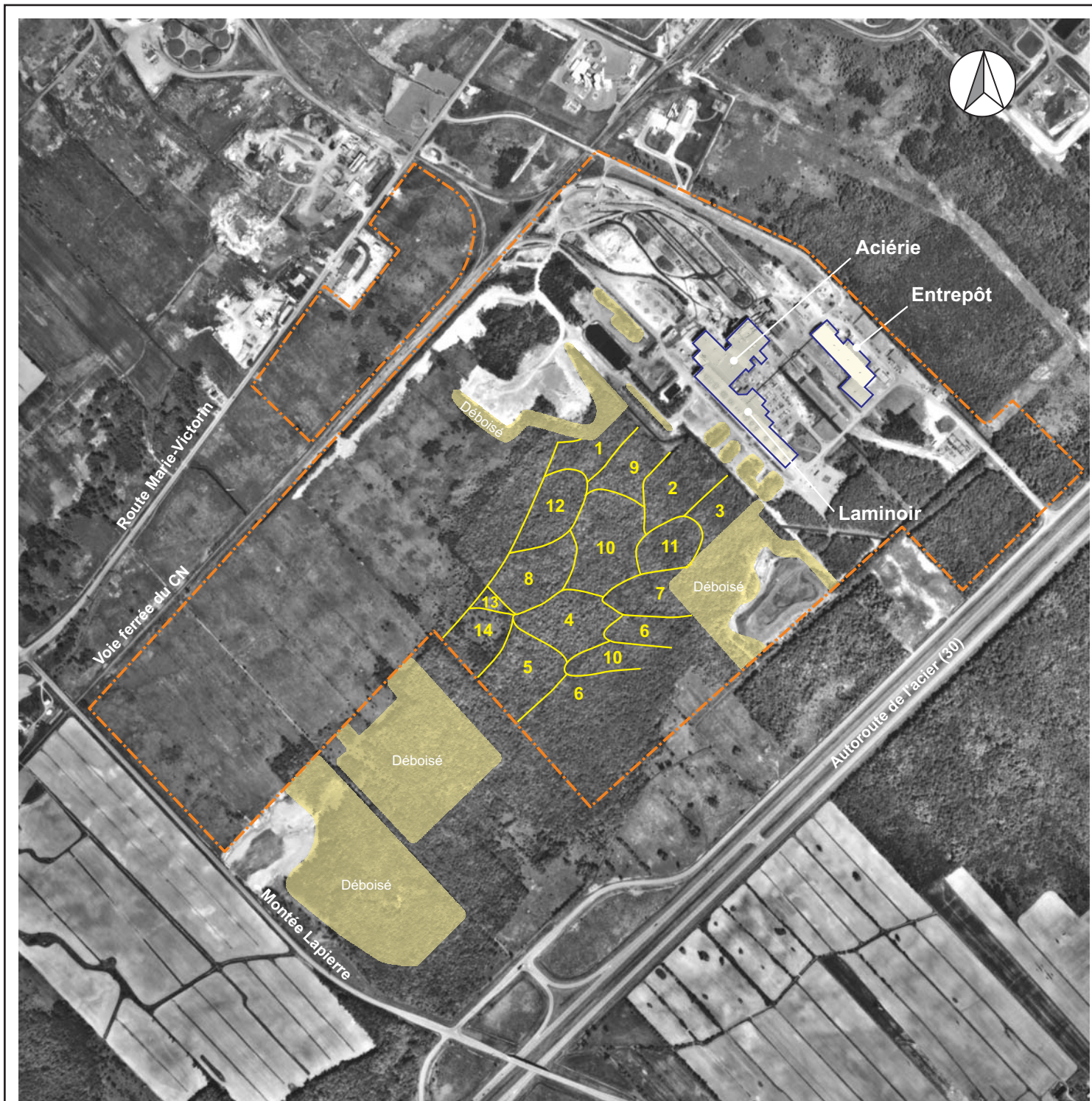
FIGURE 3-4 GROUPEMENTS VÉGÉTAUX
