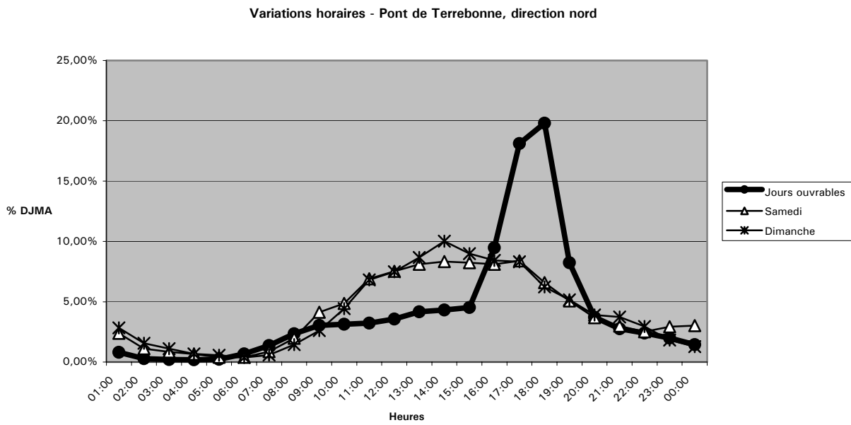
Figure 2.1 Variations horaires des débits au pont de Terrebonne par direction
