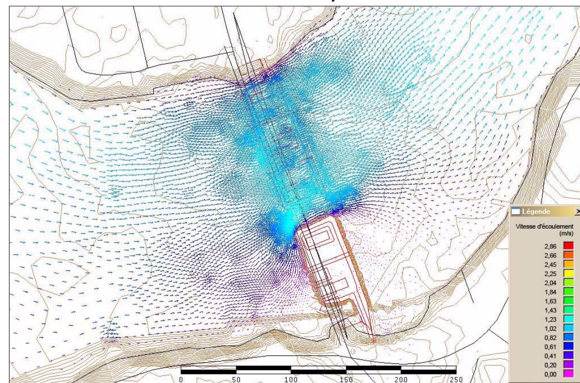
Vitesse d'écoulement – débit de 511 m 3 /s
