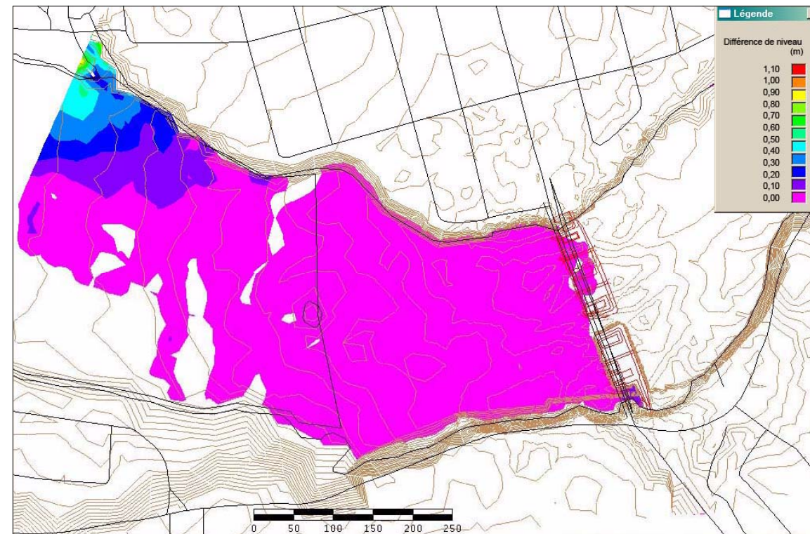
Différence de niveau – débit de 511 m 3 /s
