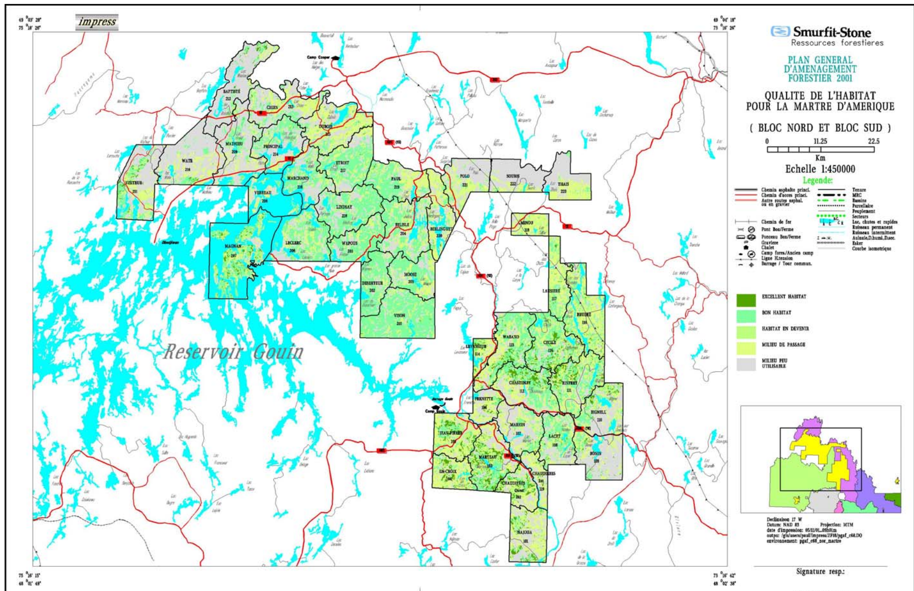
Figure 23 Qualité de l'habitat pour la martre d'Amérique
