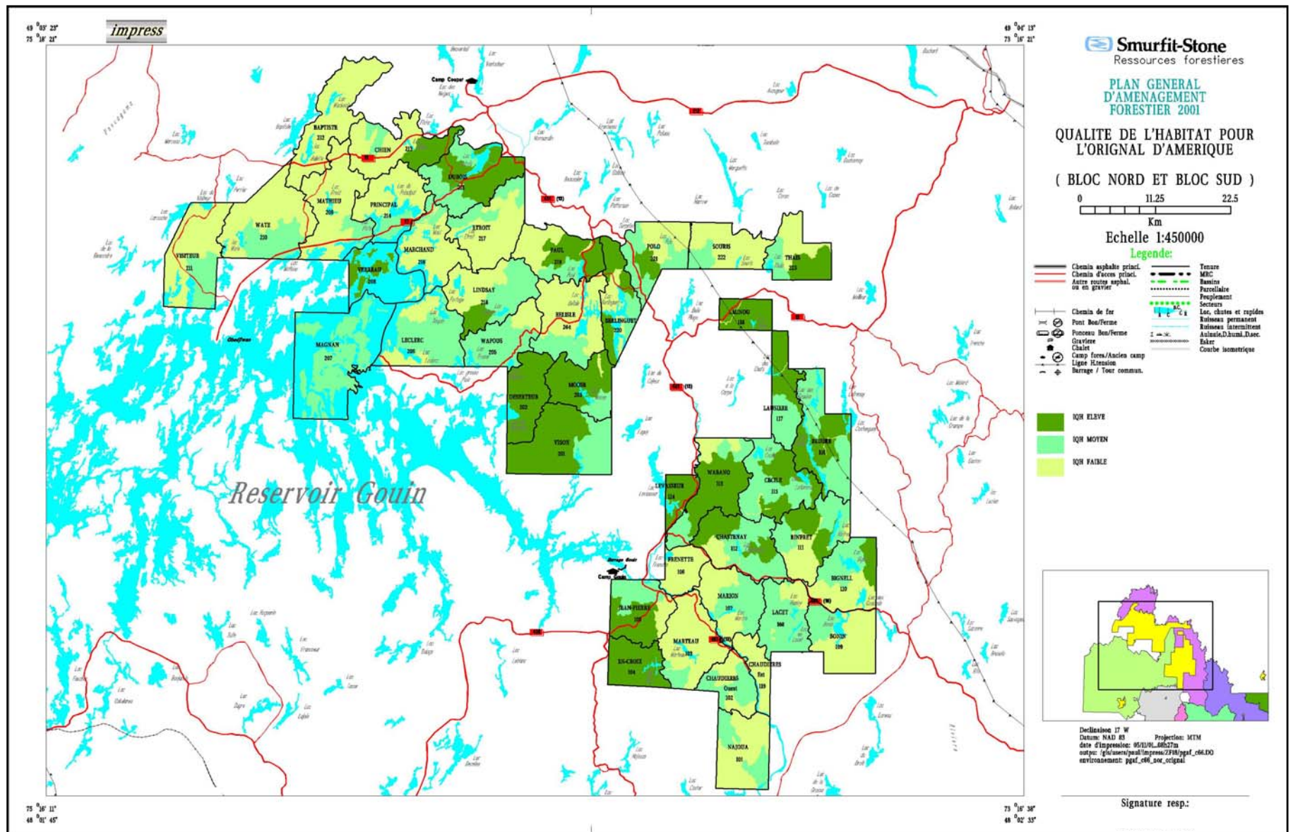
Figure 21 Qualité de l'habitat pour l'original
