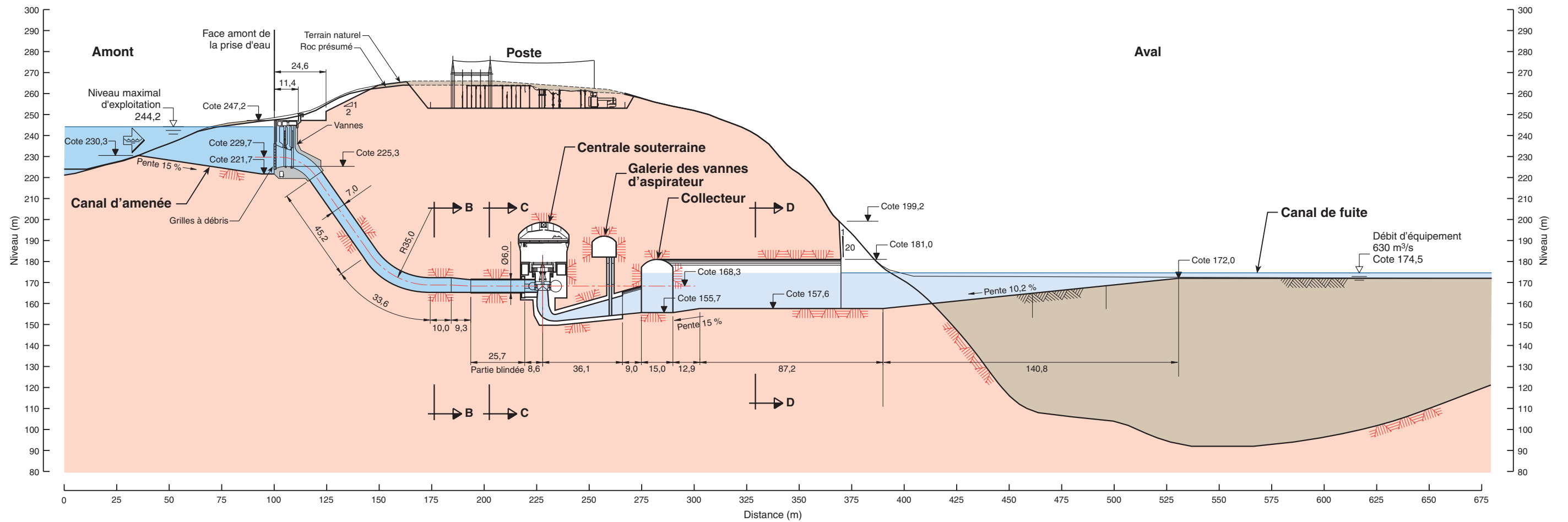
Centrale – Profil longitudinal A-A
