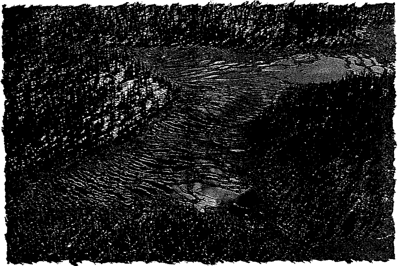
Un fen structuré près de Goose Bay (Labrador)
