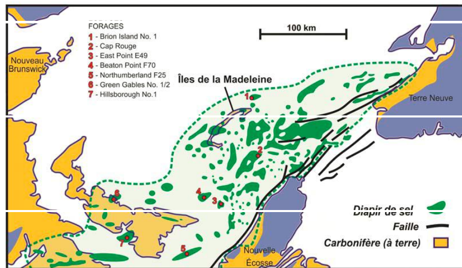
Pièges potentiels dans la zone de diapirs de sel du Bassin Madeleine. Figure tirée du document DB10, présenté par N. Pinet, de la Commission Géologique du Canada. Adaptée de Lavoie et al (2009).
