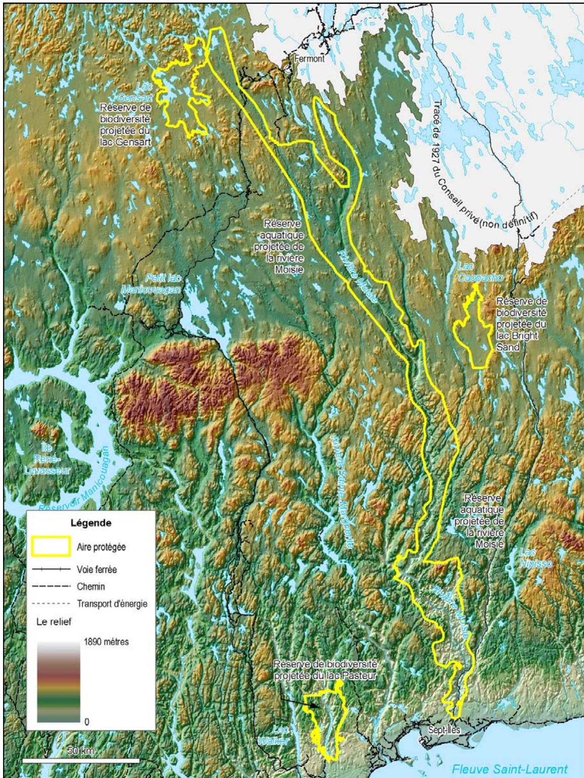
Figure 6 : Modèle numérique d'élévation (MNE) de la région
