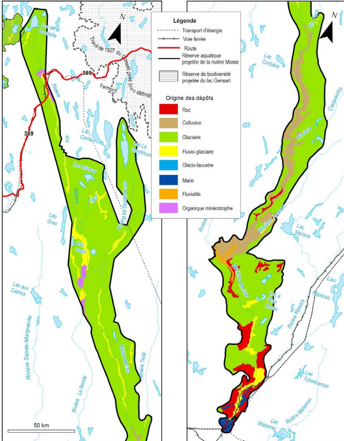
Figure 19 : Principaux dépôts de surface de la réserve aquatique projetée de la rivière Moisie
