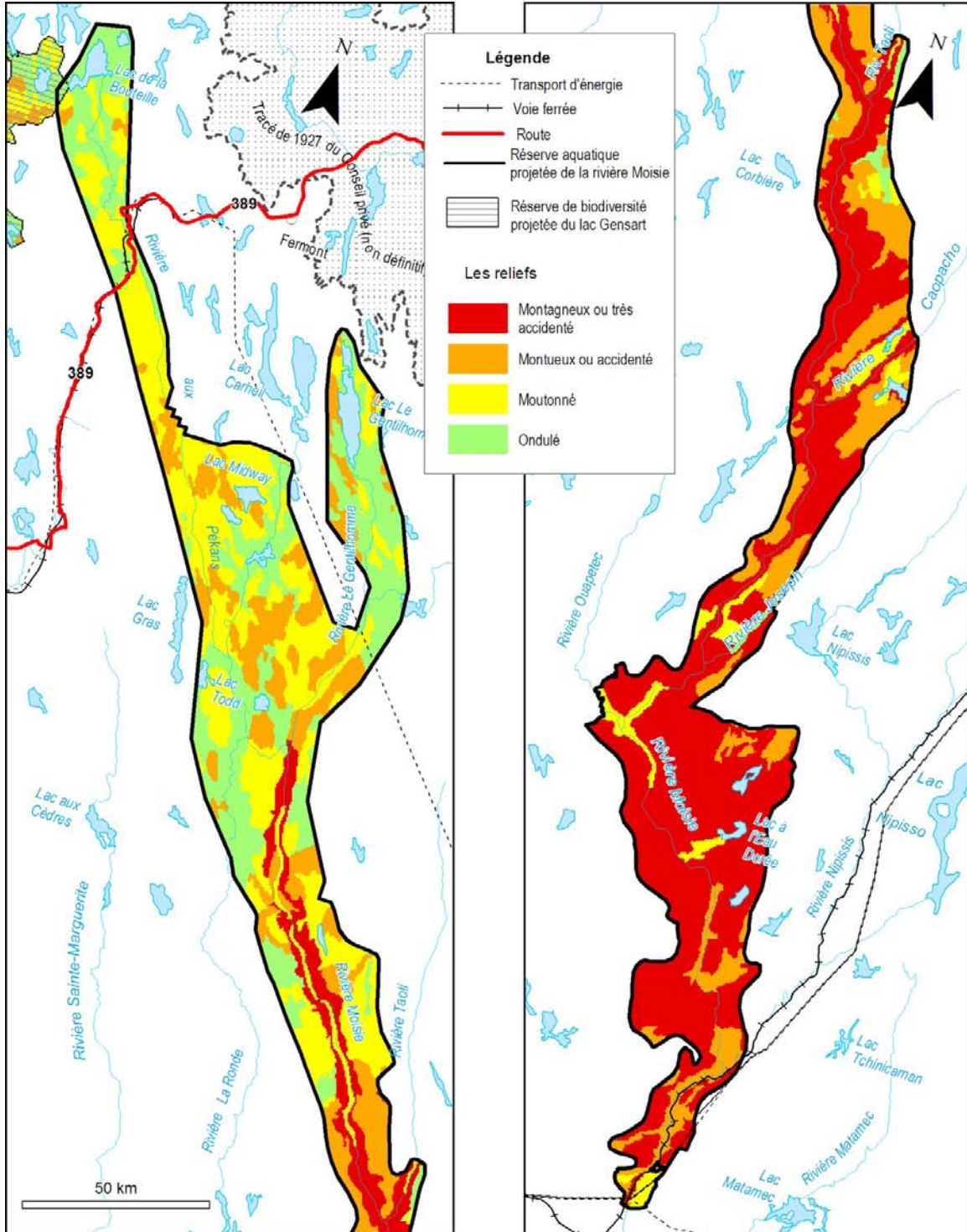
Figure 20 : Principales formes de relief de la réserve aquatique projetée de la rivière Moisie
