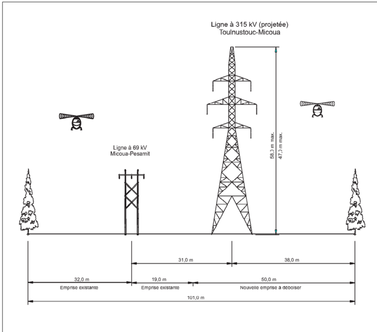
Figure 1-3 : Support et emprise types lorsque la ligne est juxtaposée à une ligne existante
