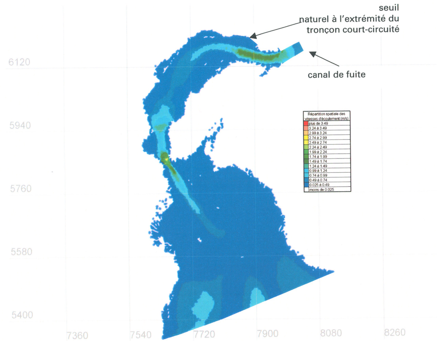
Figure RQC-9.17b Répartition des vitesses d'écoulement, en conditions futures caractéristiques du mois d'octobre, débit de la rivière Magpie de 187 m 3 /s, dont 184 m 3 /s turbinés et 3 m 3 /s en guise de débit réservé écologique (conditions de marée haute)
