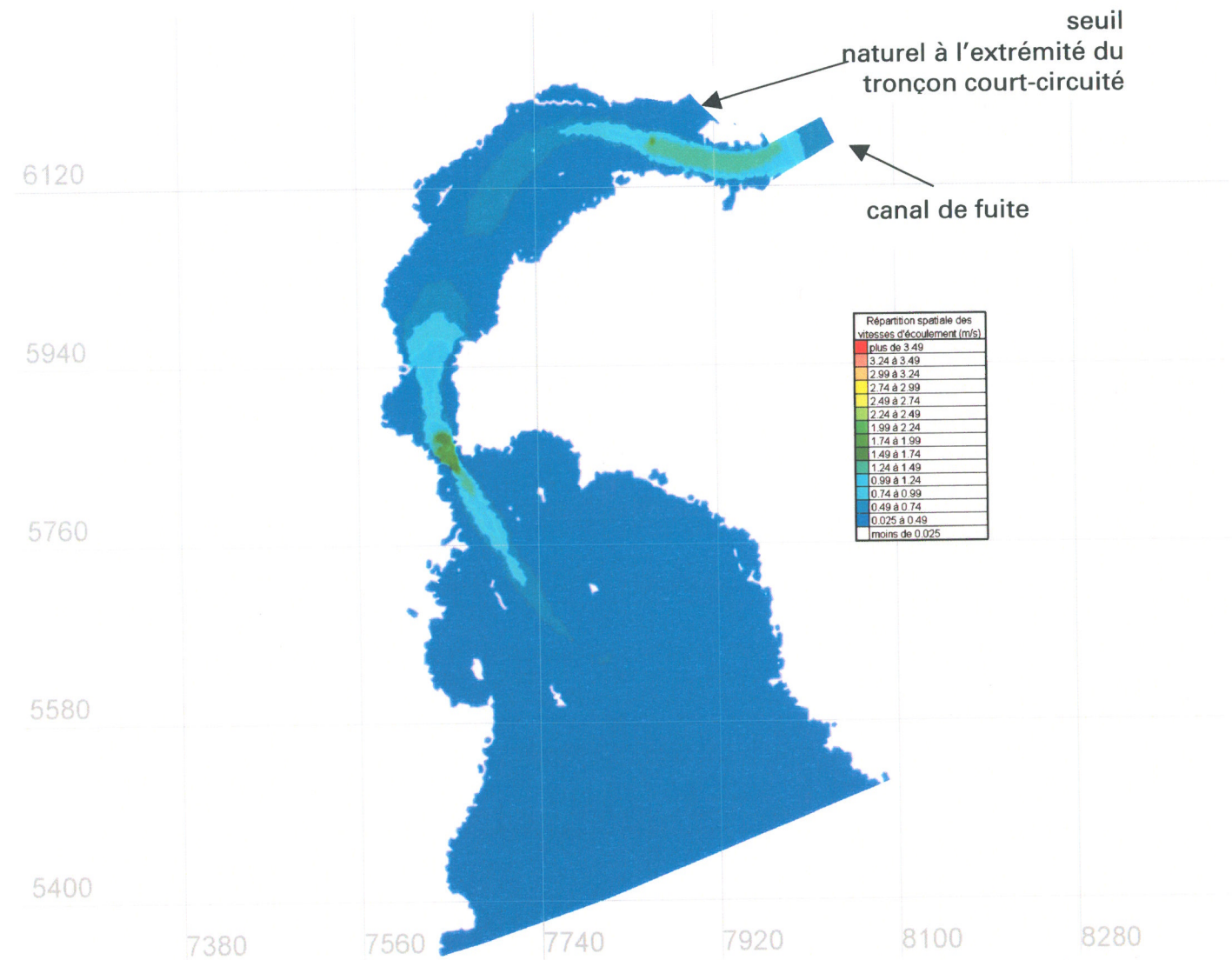
Figure RQC-9.16b Répartition des vitesses d'écoulement, en conditions futures caractéristiques du mois de septembre, débit de la rivière Magpie de 164 m 3 /s, dont 161 m 3 /s turbinés et 3 m 3 /s en guise de débit réservé écologique (conditions de marée haute)
