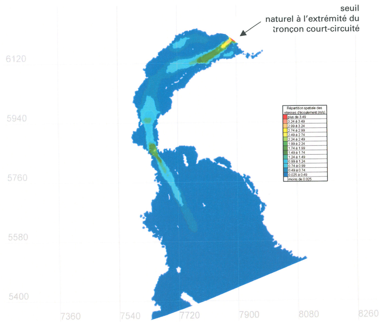
Figure RQC-9.17a Répartition spatiale des vitesses d'écoulement, en conditions actuelles caractéristiques du mois d'octobre, débit de la rivière Magpie de 187 m 3 /s (conditions de marée haute)
