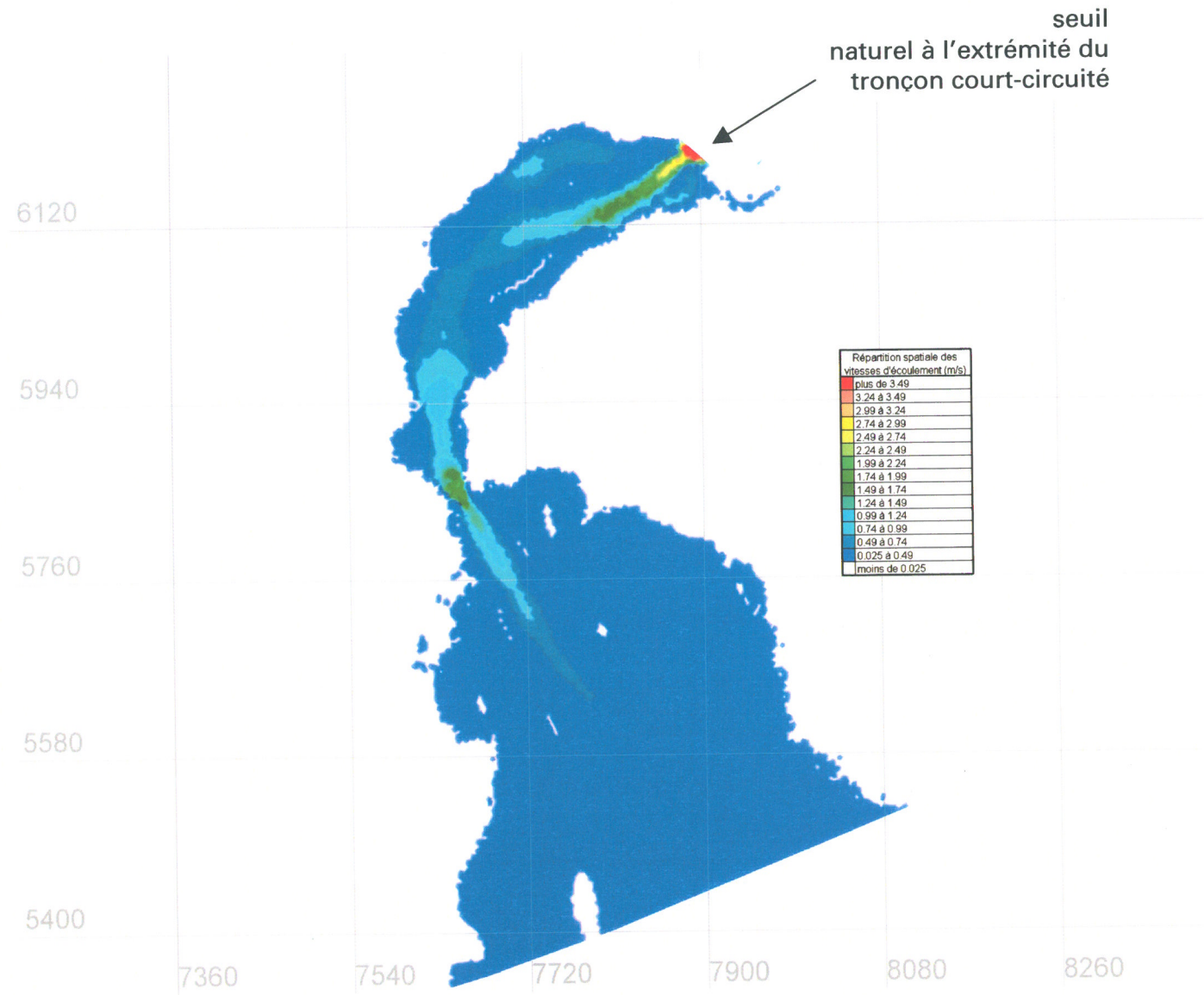
Figure RQC-9.16a Répartition spatiale des vitesses d'écoulement, en conditions actuelles caractéristiques du mois de septembre, débit de la rivière Magpie de 164 m 3 /s (conditions de marée haute)
