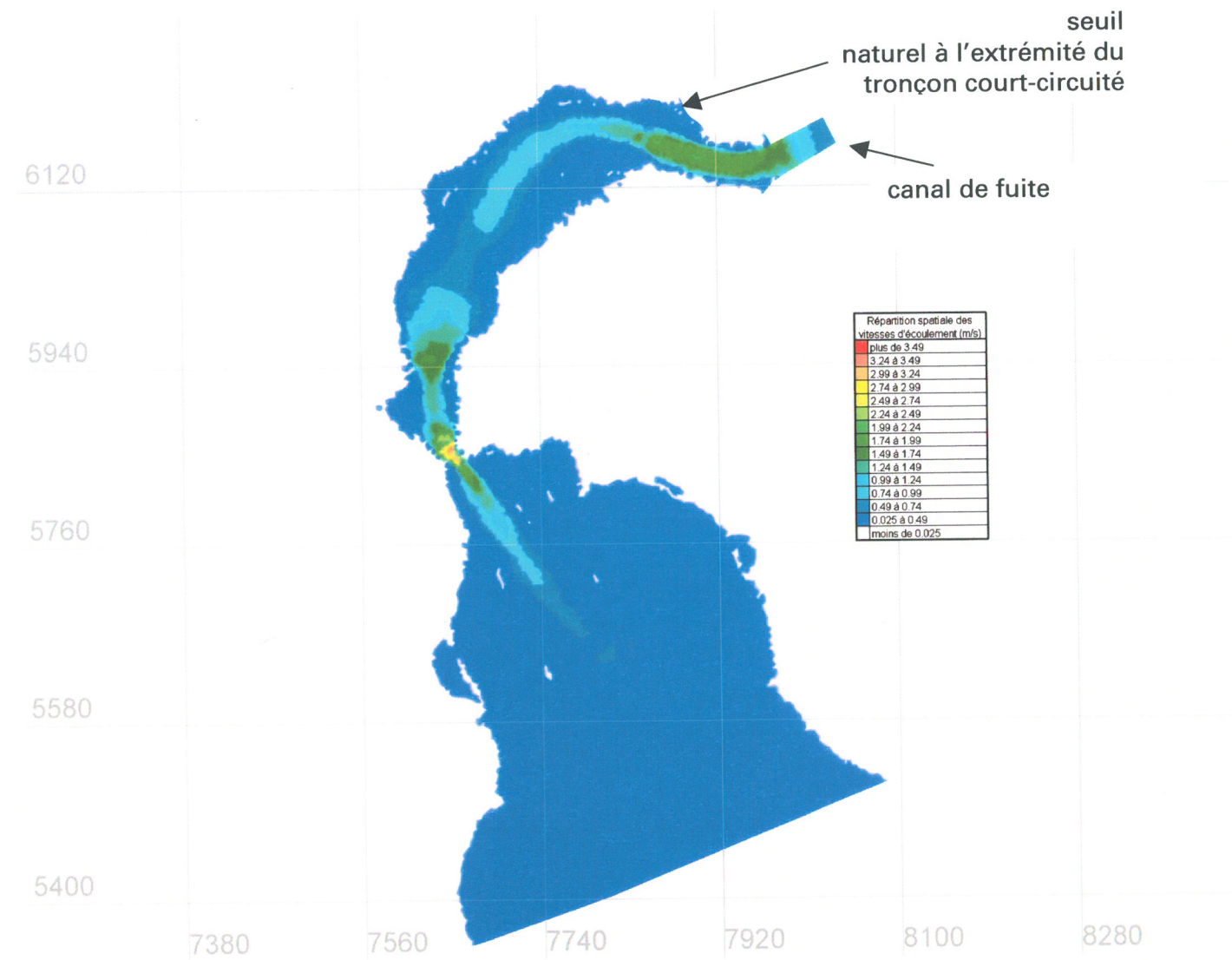
Figure RQC-9.12b Répartition des vitesses d'écoulement, en conditions futures caractéristiques du mois d'octobre, débit de la rivière Magpie de 187 m 3 /s, dont 184 m 3 /s turbinés et 3 m 3 /s en guise de débit réservé écologique (conditions de marée moyenne)
