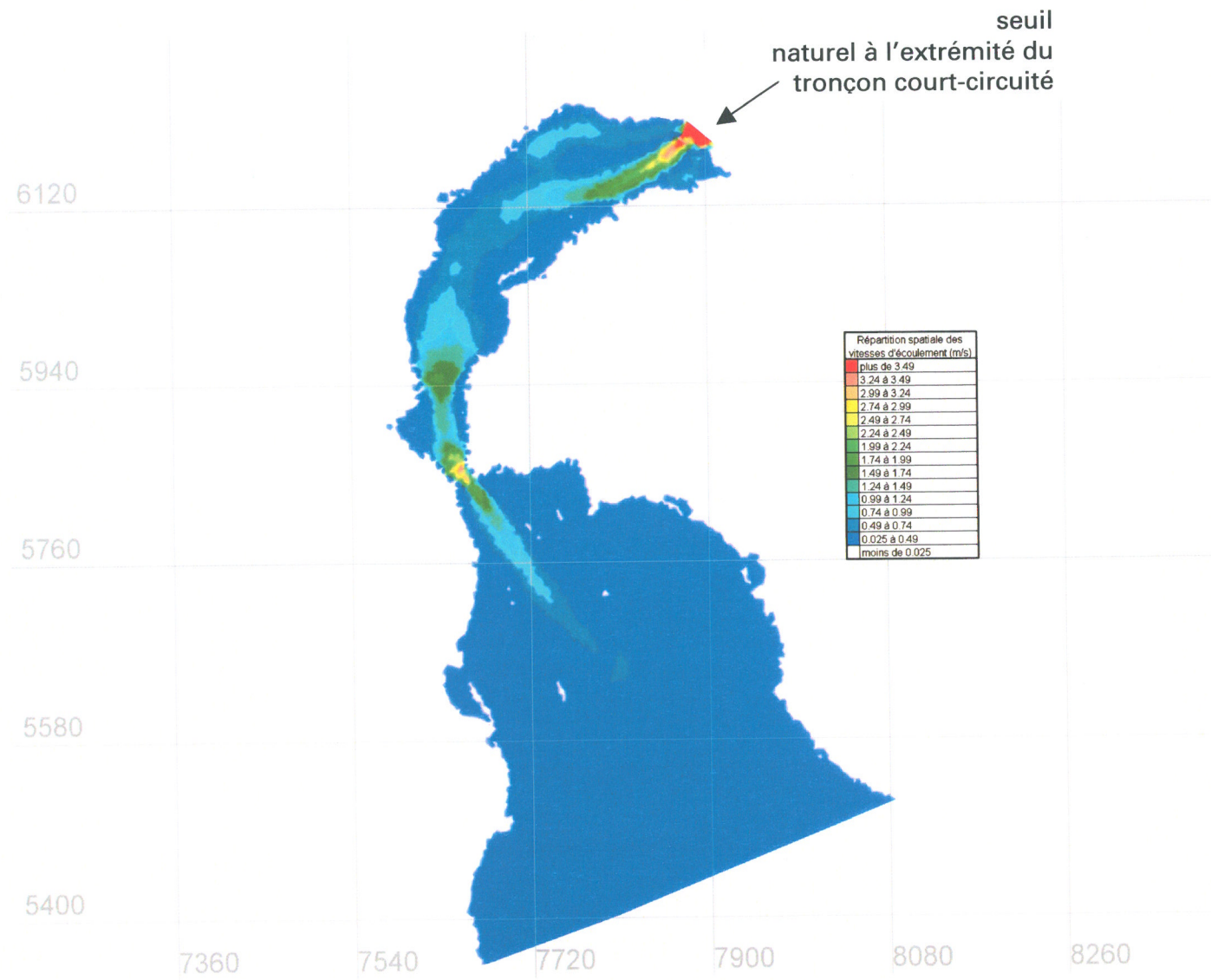
Figure RQC-9.12a Répartition spatiale des vitesses d'écoulement, en conditions actuelles caractéristiques du mois d'octobre, débit de la rivière Magpie de 187 m 3 /s (conditions de marée moyenne)
