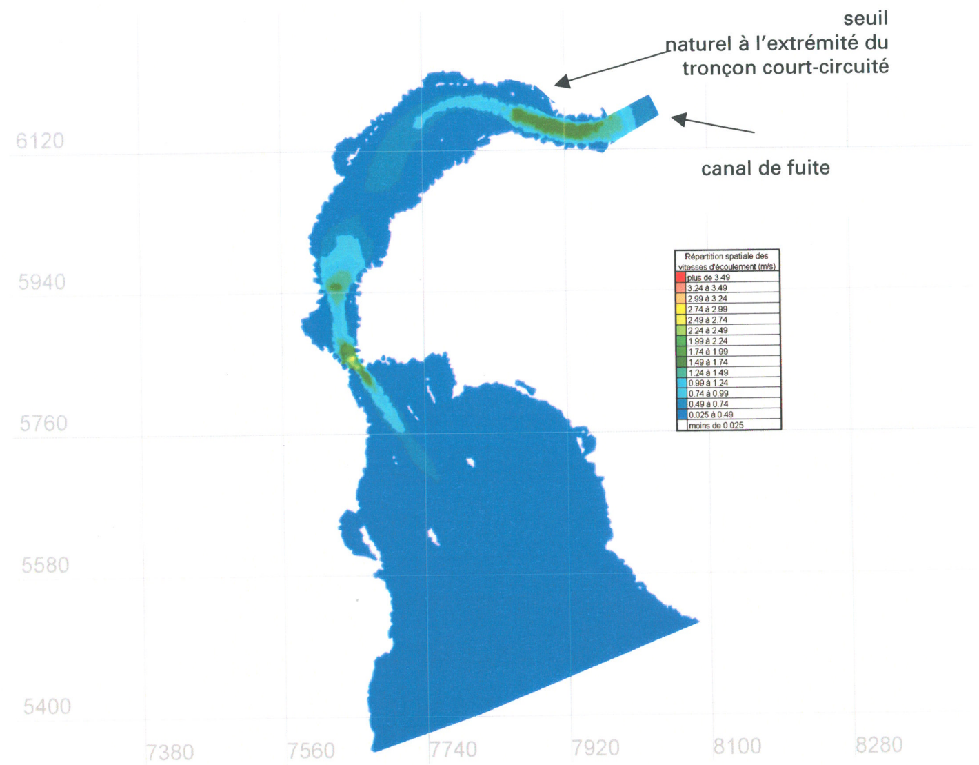
Figure RQC-9.13b Répartition des vitesses d'écoulement, en conditions futures caractéristiques du mois de novembre, débit de la rivière Magpie de 146 m 3 /s, dont 143 m 3 /s turbinés et 3 m 3 /s en guise de débit réservé écologique (conditions de marée moyenne)
