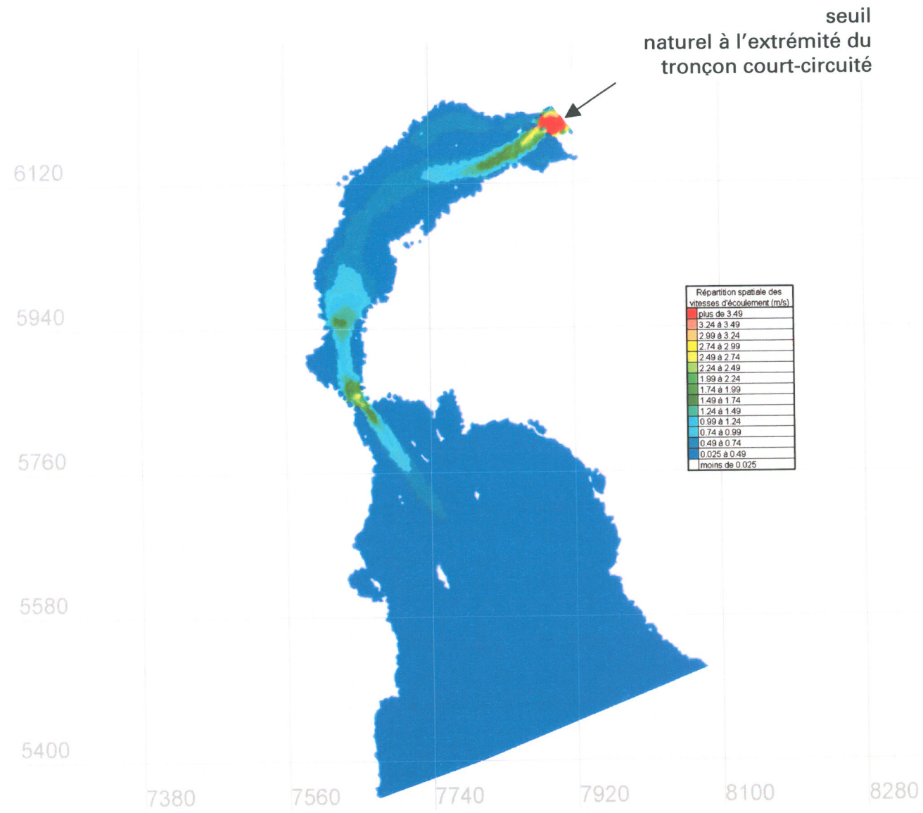
Figure RQC-9.13a Répartition spatiale des vitesses d'écoulement, en conditions actuelles caractéristiques du mois de novembre, débit de la rivière Magpie de 146 m 3 /s (conditions de marée moyenne)
