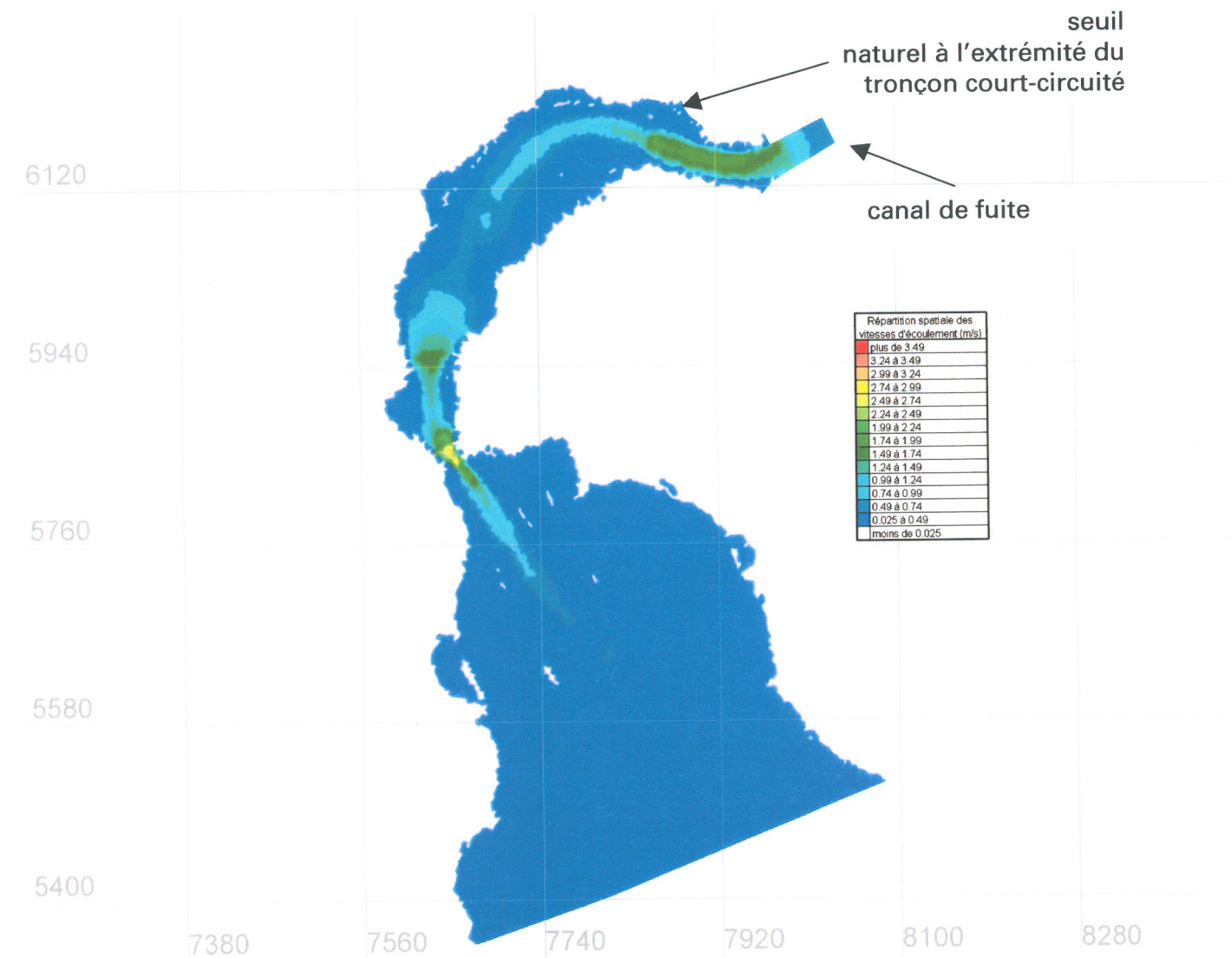
Figure RQC-9.11b Répartition des vitesses d'écoulement, en conditions futures caractéristiques du mois de septembre, débit de la rivière Magpie de 164 m 3 /s, dont 161 m 3 /s turbinés et 3 m 3 /s en guise de débit réservé écologique (conditions de marée moyenne)
