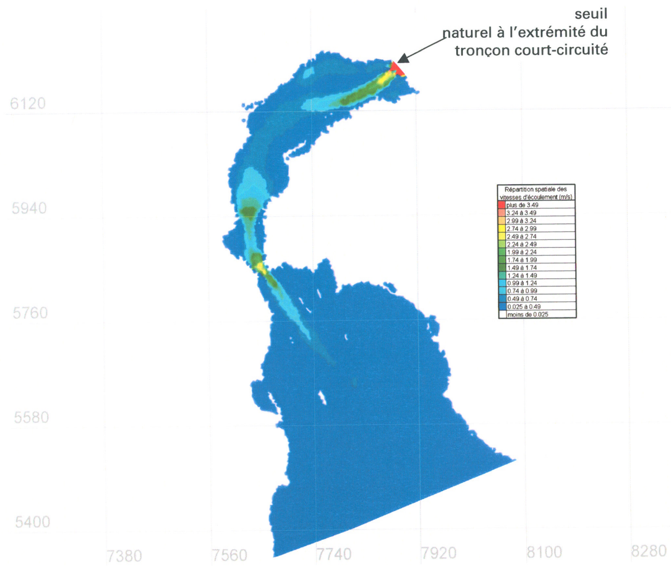
Figure RQC-9.11a Répartition spatiale des vitesses d'écoulement, en conditions actuelles caractéristiques du mois de septembre, débit de la rivière Magpie de 164 m 3 /s (conditions de marée moyenne)
