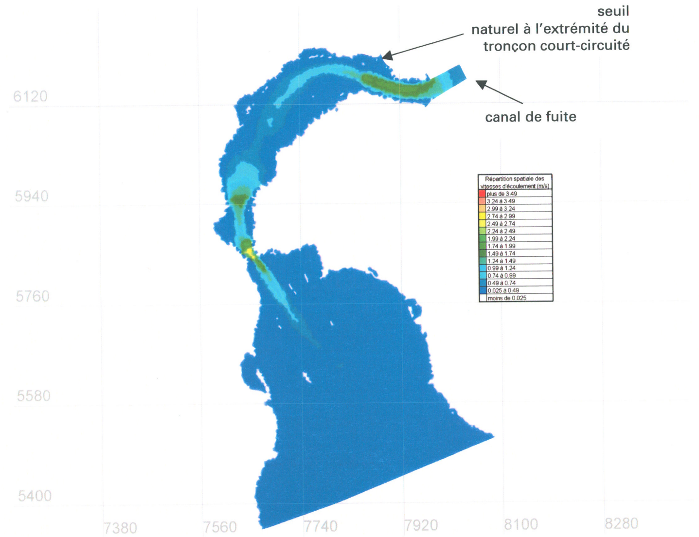
Figure RQC-9.10b Répartition des vitesses d'écoulement, en conditions futures caractéristiques du mois d'août, débit de la rivière Magpie de 161 m 3 /s, dont 158 m 3 /s turbinés et 3 m 3 /s en guise de débit réservé écologique (conditions de marée moyenne)
