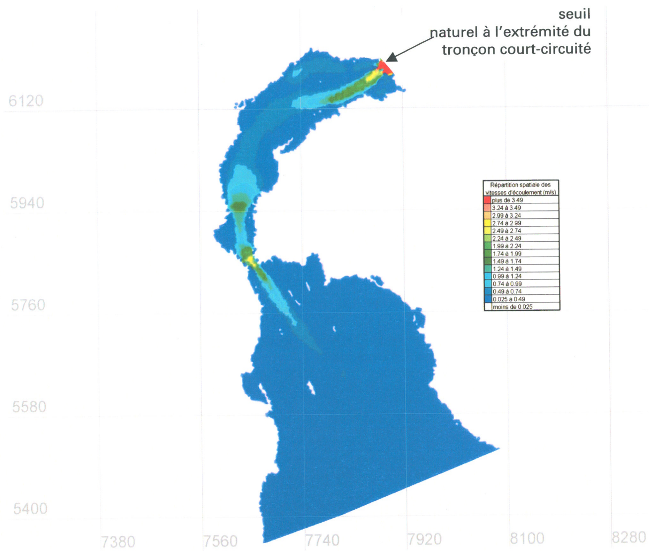
Figure RQC-9.10a Répartition spatiale des vitesses d'écoulement, en conditions actuelles caractéristiques du mois d'août, débit de la rivière Magpie de 161 m 3 /s (conditions de marée moyenne)
