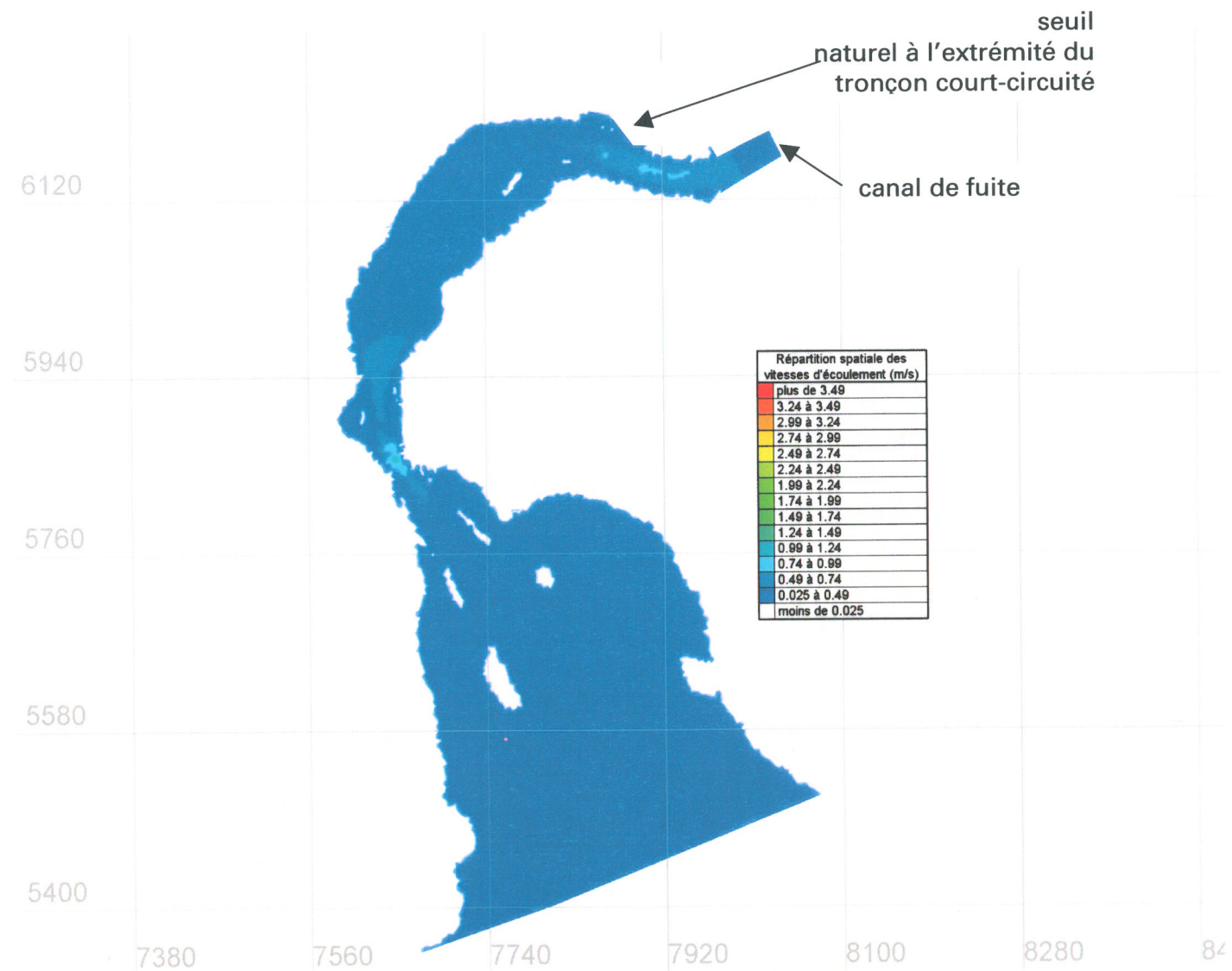
Figure RQC-9.1b Répartition spatiale des vitesses d'écoulement, en conditions futures caractéristiques du mois de janvier, débit de la rivière Magpie de 59 m 3 /s, dont 56 m 3 /s turbinés et 3 m 3 /s en guise de débit écologique (conditions de marée moyenne)
