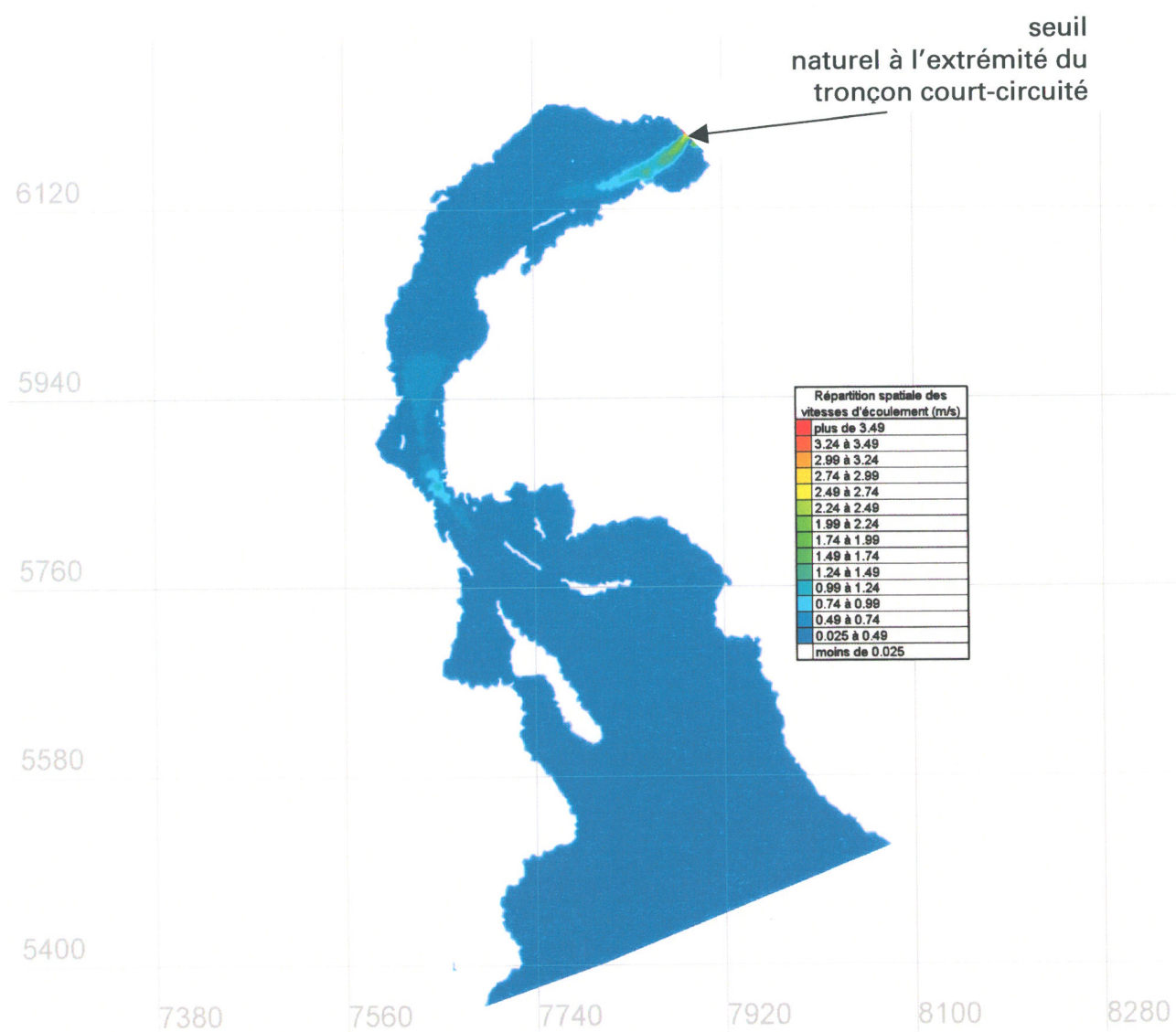
Figure RQC-9.1a Répartition spatiale des vitesses d'écoulement, en conditions actuelles caractéristiques du mois de janvier, débit de la rivière Magpie de 59 m 3 /s (conditions de marée moyenne)
