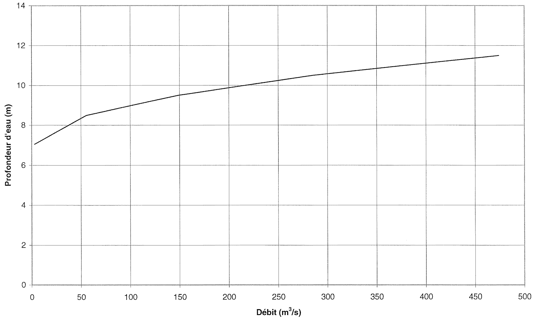
Figure RQC-7.2 Profondeur d'écoulement maximal en fonction du débit le long du tronçon court-circuité
