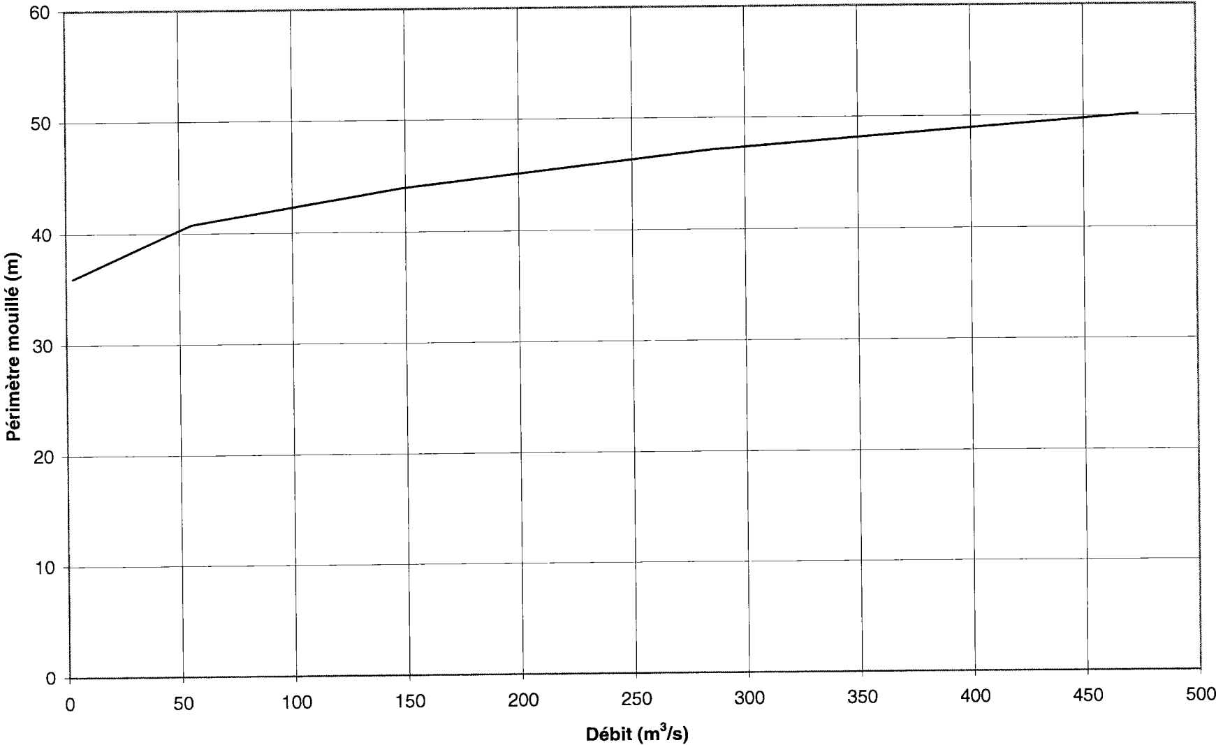
Figure RQC-7.1 Périmètre mouillé en fonction du débit, tronçon court-circuité
