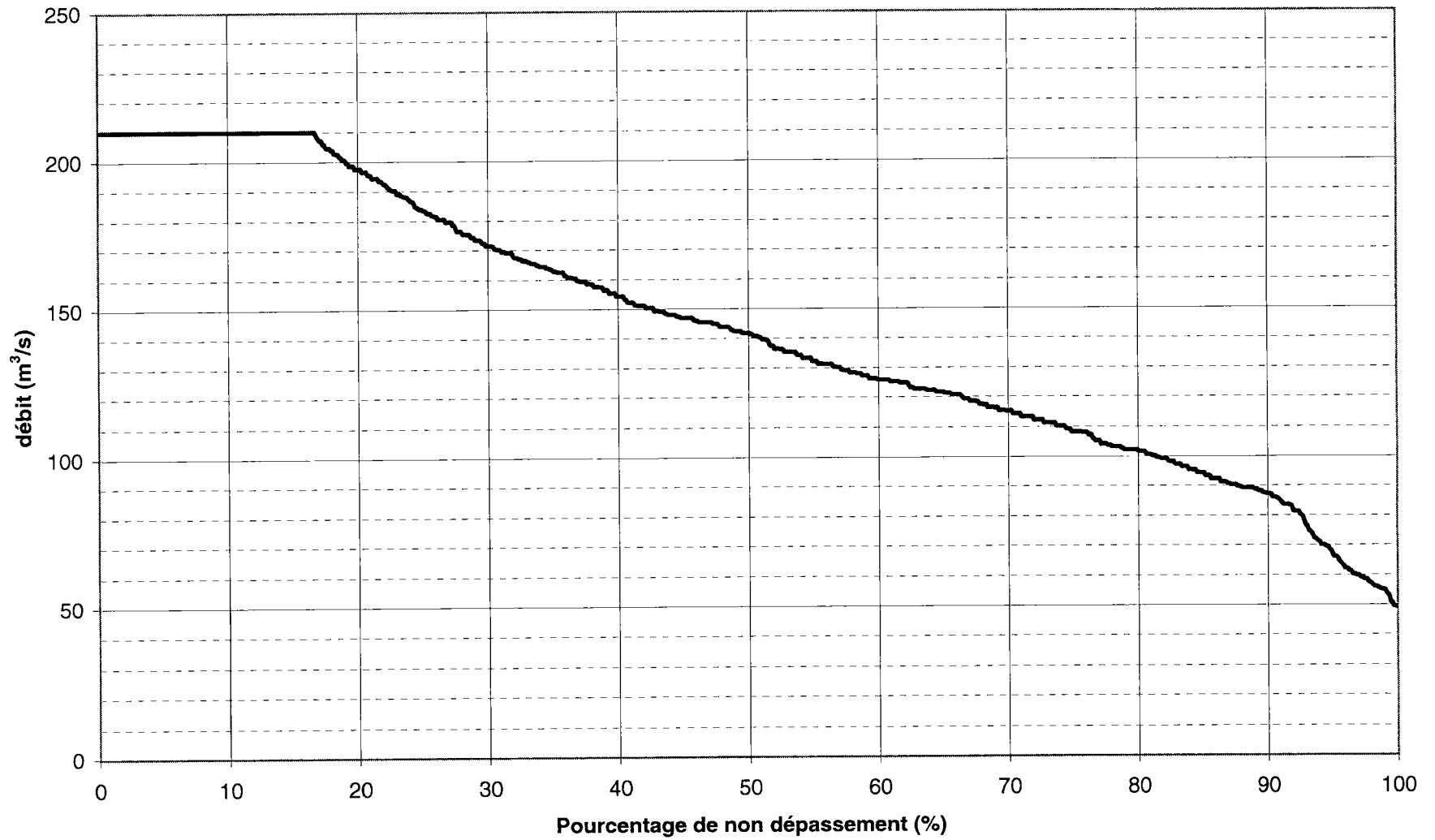
Figure RQC-4.3 Courbe des débits turbinés classés caractéristiques de la période de montaison des anguilles - août
