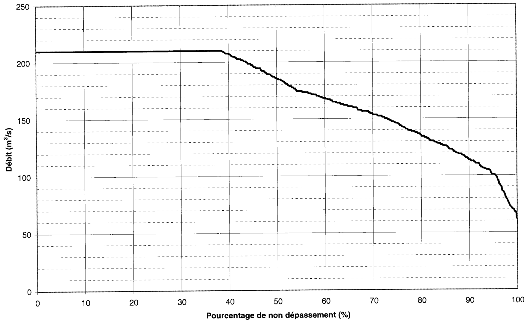
Figure RQC-4.2 Courbe des débits turbinés classés caractéristiques de la période de montaison des anguilles - juillet
