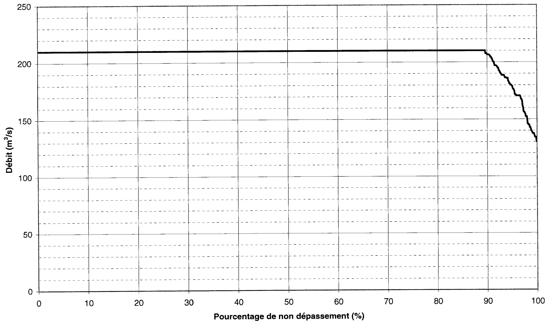
Figure RQC-4.1 Courbe des débits turbinés classés caractéristiques de la période de montaison des anguilles - juin
