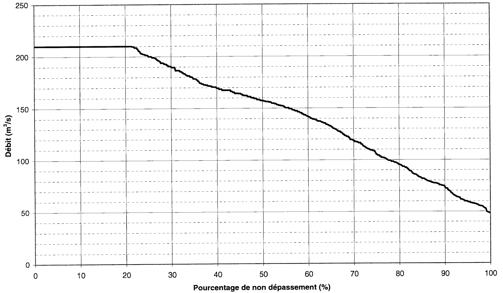
Figure RQC-4.4 Courbe des débits turbinés classés caractéristiques de la période de montaison des anguilles - septembre
