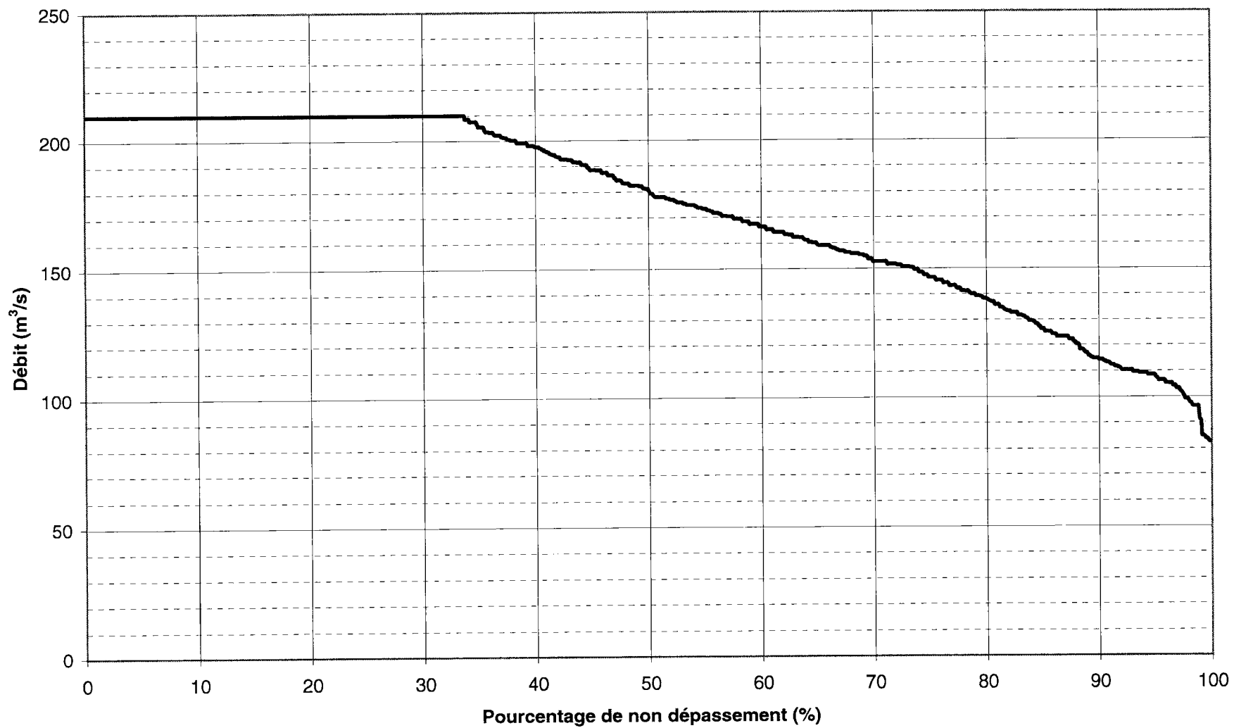
Figure RQC-4.5 Courbe des débits turbinés classés caractéristiques de la période de montaison des anguilles - octobre
