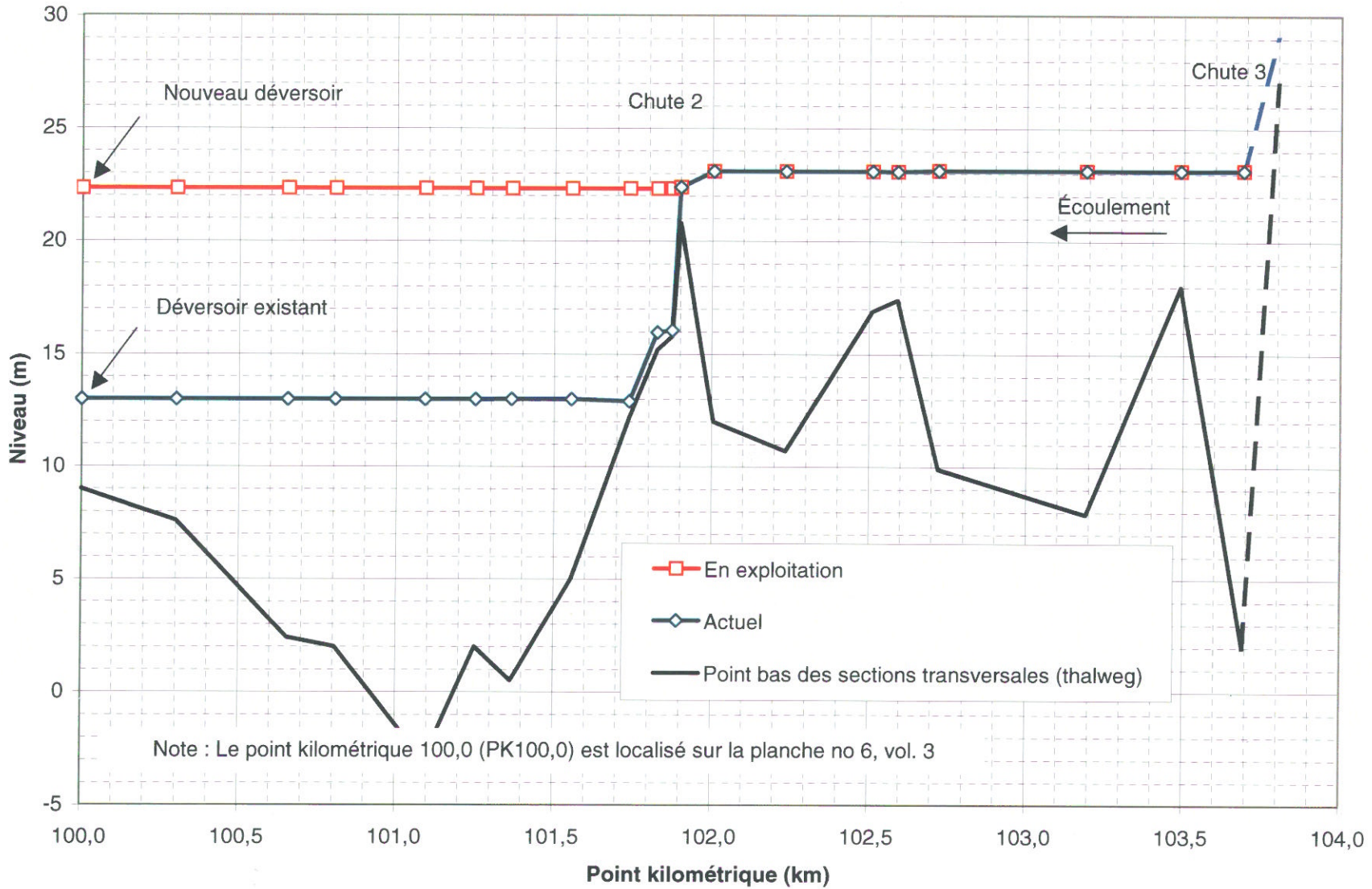
Figure 8.1 Profil de la surface libre le long du tronçon amont en étiage estival ( Q_{2-7} 108 \text{ m}^3/\text{s} )
