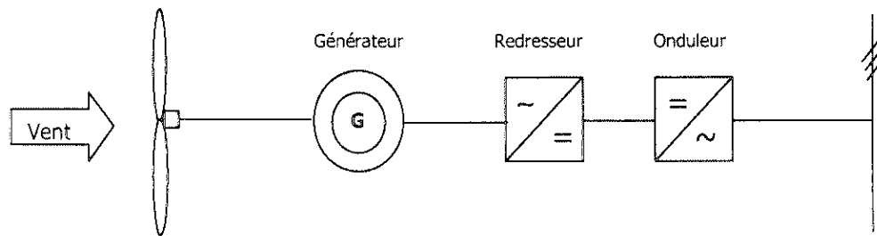
Figure 2.6 : Chaîne de conversion d'une éolienne à vitesse variable
