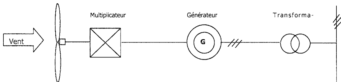
Figure 2.4 : Chaîne de conversion d'une éolienne à vitesse fixe
