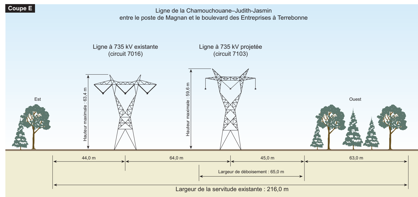
Figure 3 : Supports et emprises types de la ligne et de la déviation projetées – Coupes E à H
