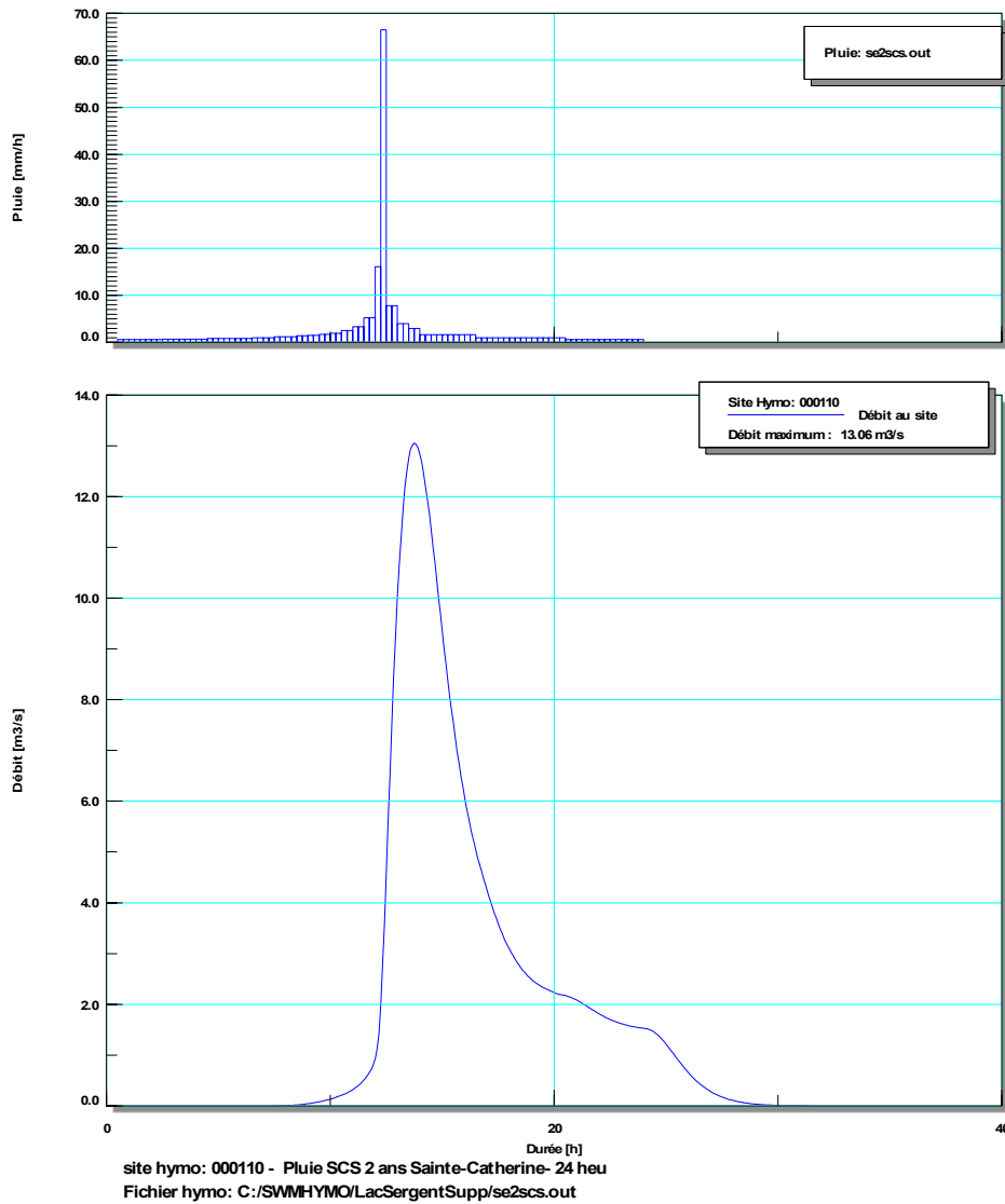
Hydrogramme d'entrée 1/2 ans
