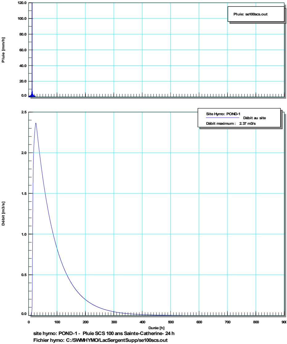
Hydrogramme de sortie 1/100 ans
