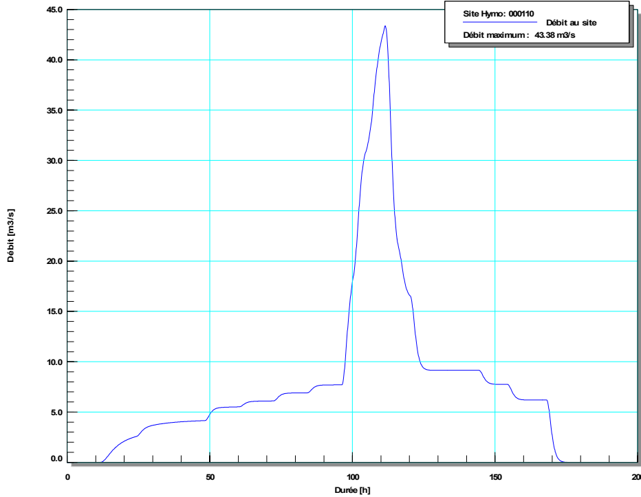
Hydrogramme d'entrée 1/100 ans
