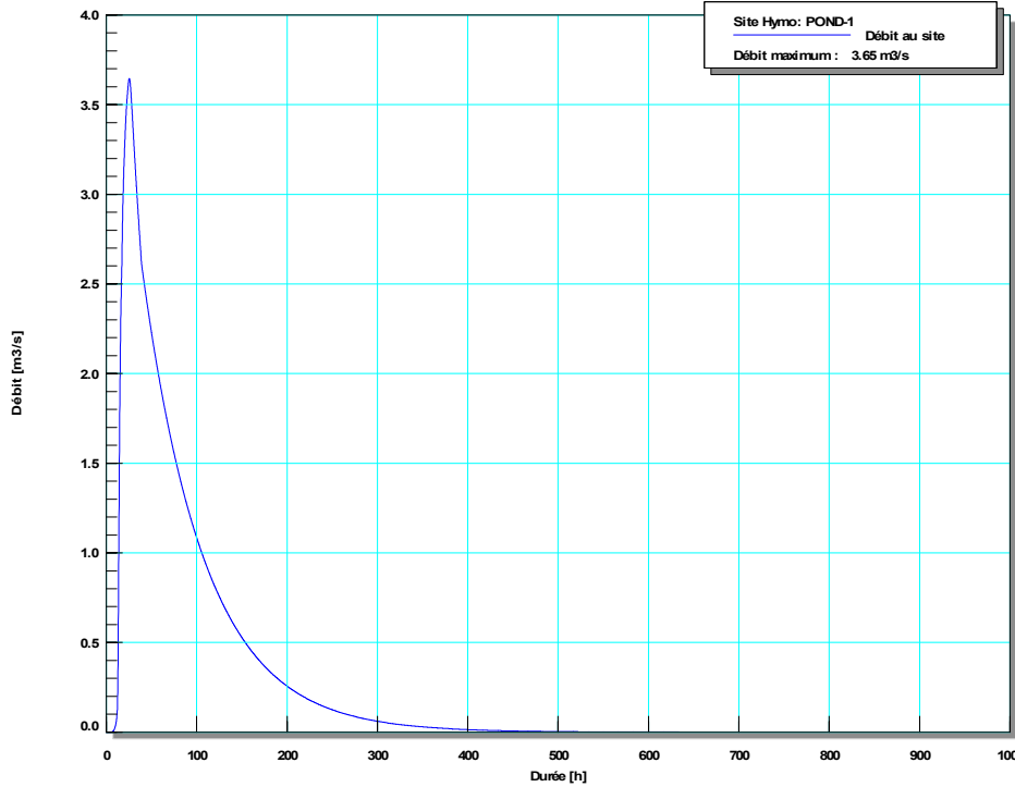
Hydrogramme de sortie 1/1000 ans
