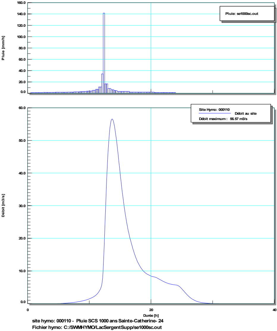
Hydrogramme d'entrée 1/1000 ans
