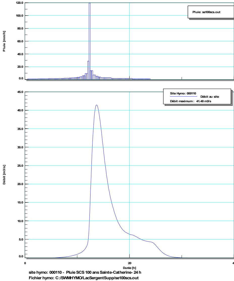
Hydrogramme d'entrée 1/100 ans
