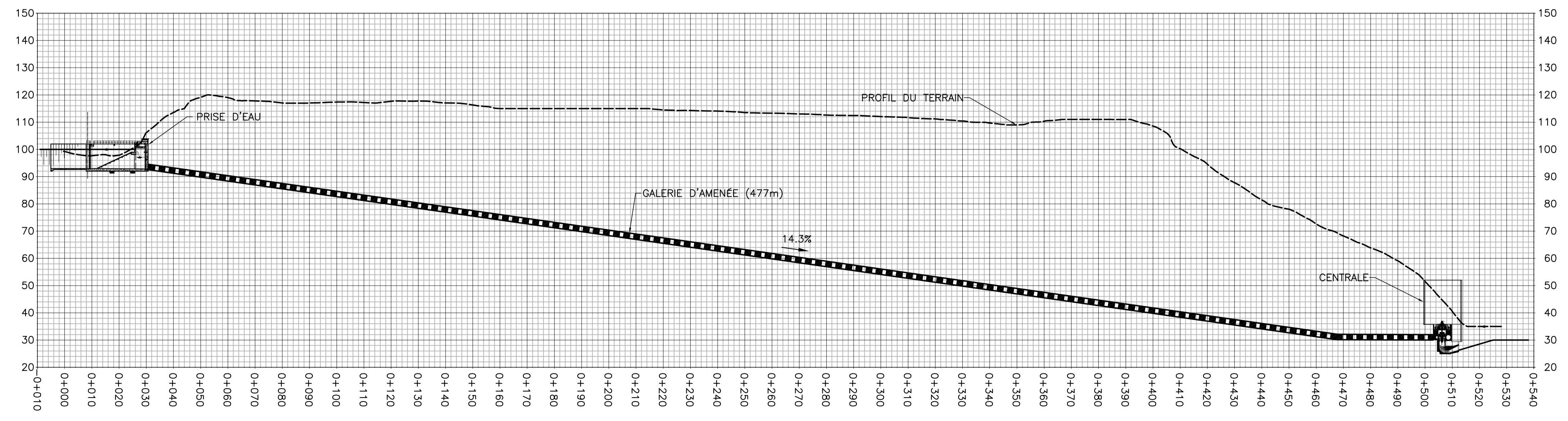
COUPE 1 ÉCH. 1:300
