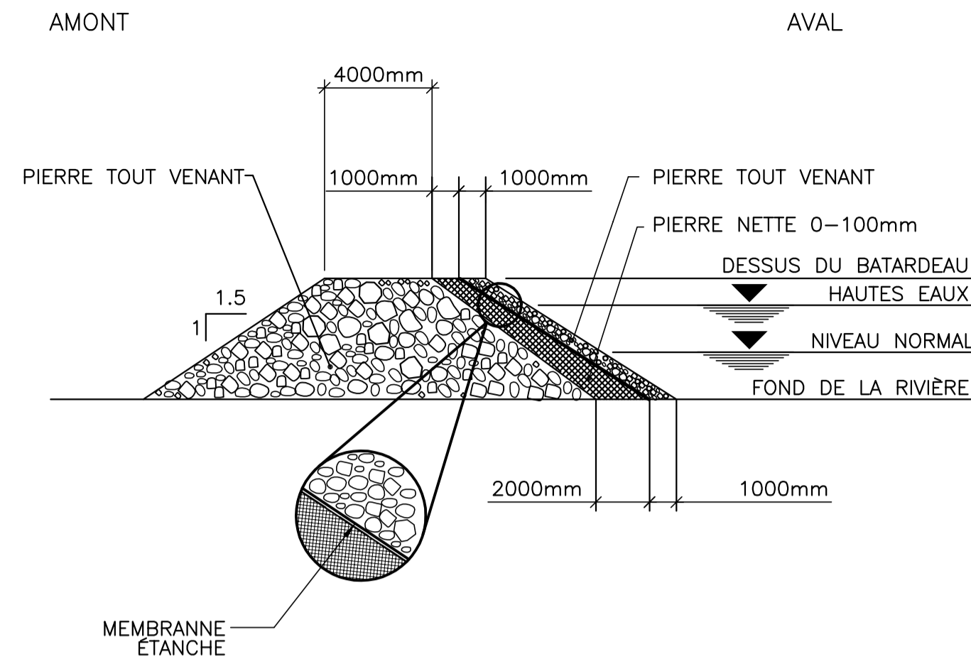
BATARDEAU - AVAL SECTION TYPE ECH. AUCUNE
