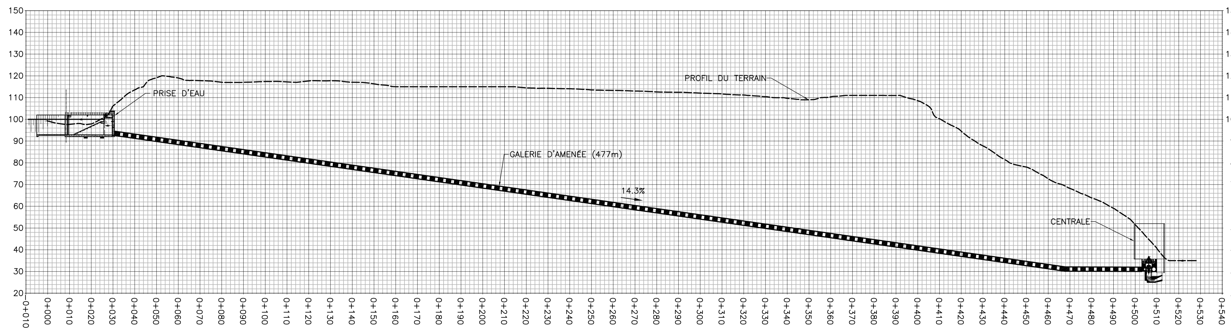
COUPE ① ÉCH. 1:300
