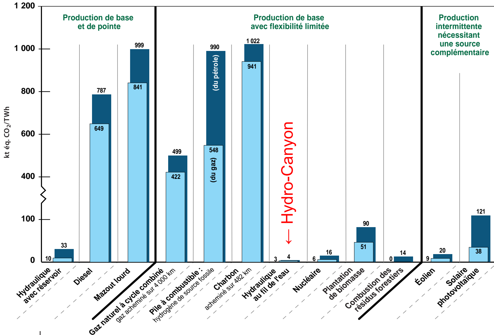
Figure 1 – Émissions de gaz à effet de serre (kt éq. CO 2 /TWh)
