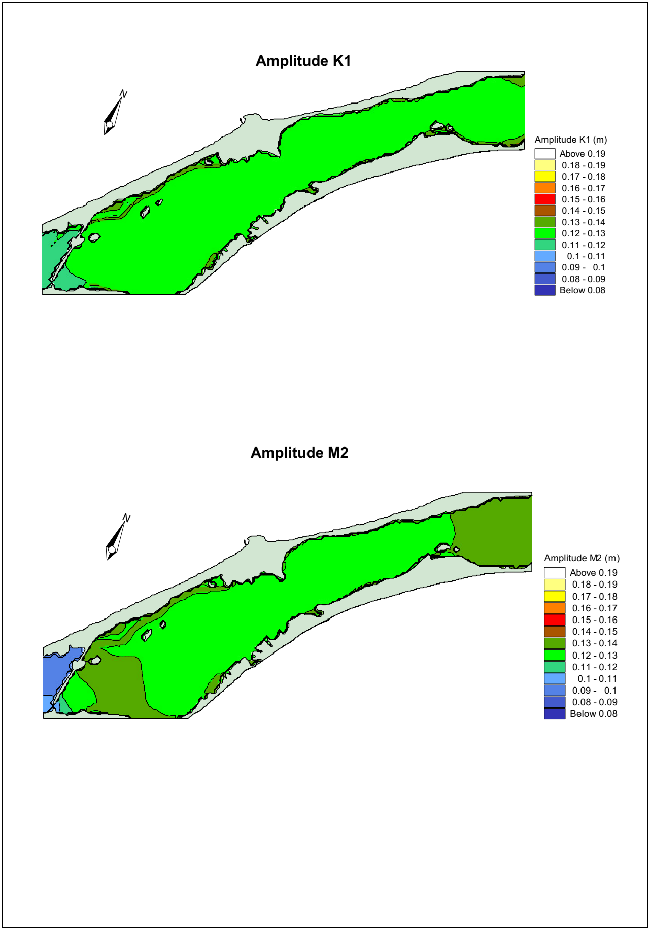
Annexe 3.3 Amplitude des composantes harmoniques diurne (K1) et semi-diurne (M2) dans la lagune de la Grande Entrée.
