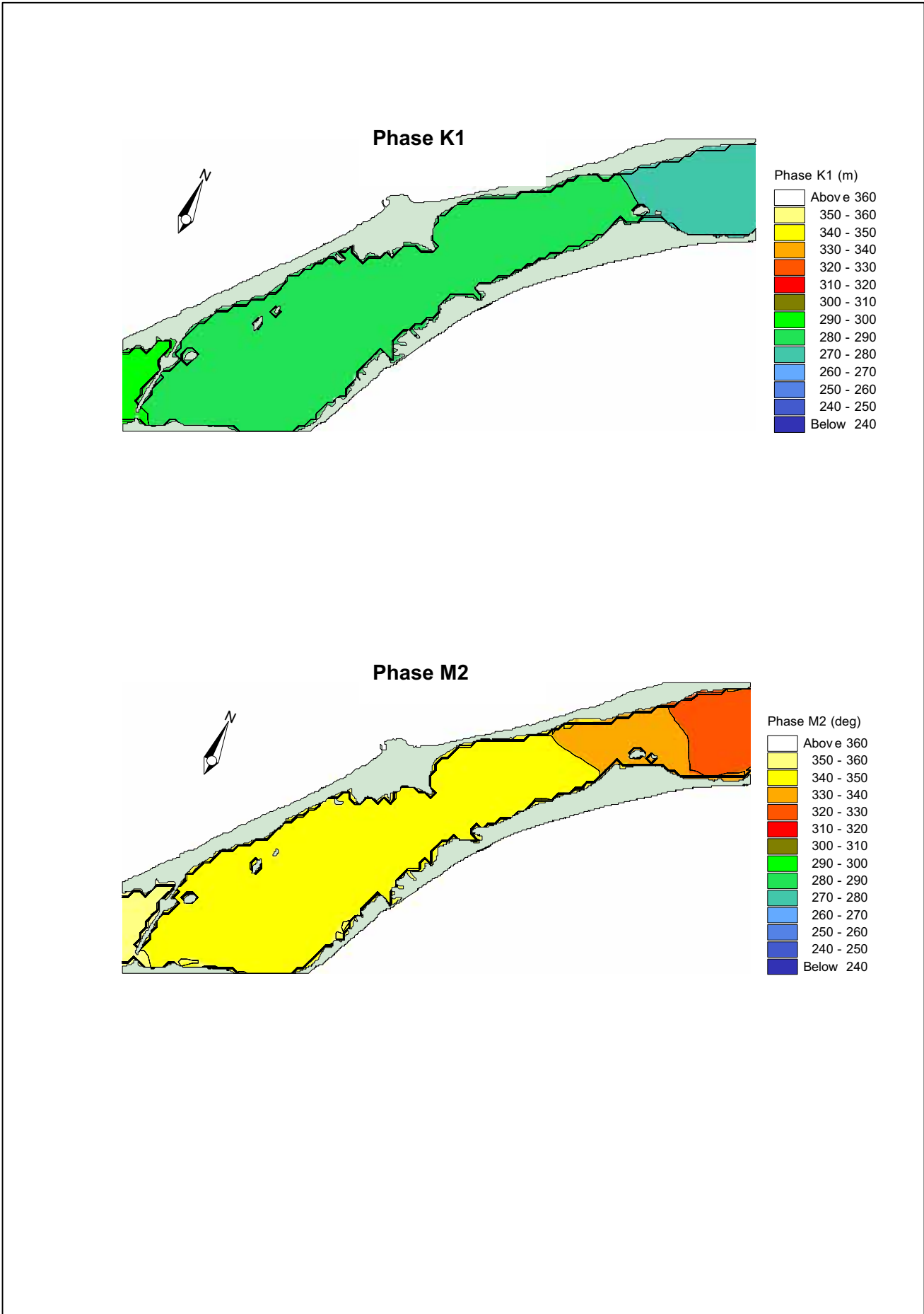
Annexe 3.4 Phase des composantes harmoniques diurne (K1) et semi-diurne (M2) dans la lagune de la Grande Entrée.
