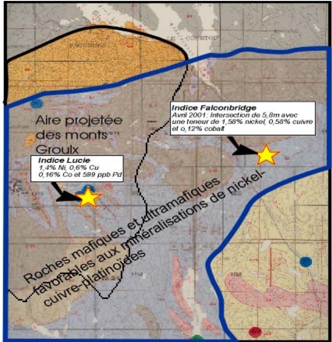
Limite de l'Aire protégée des Monts Groulx et géologie régionale
