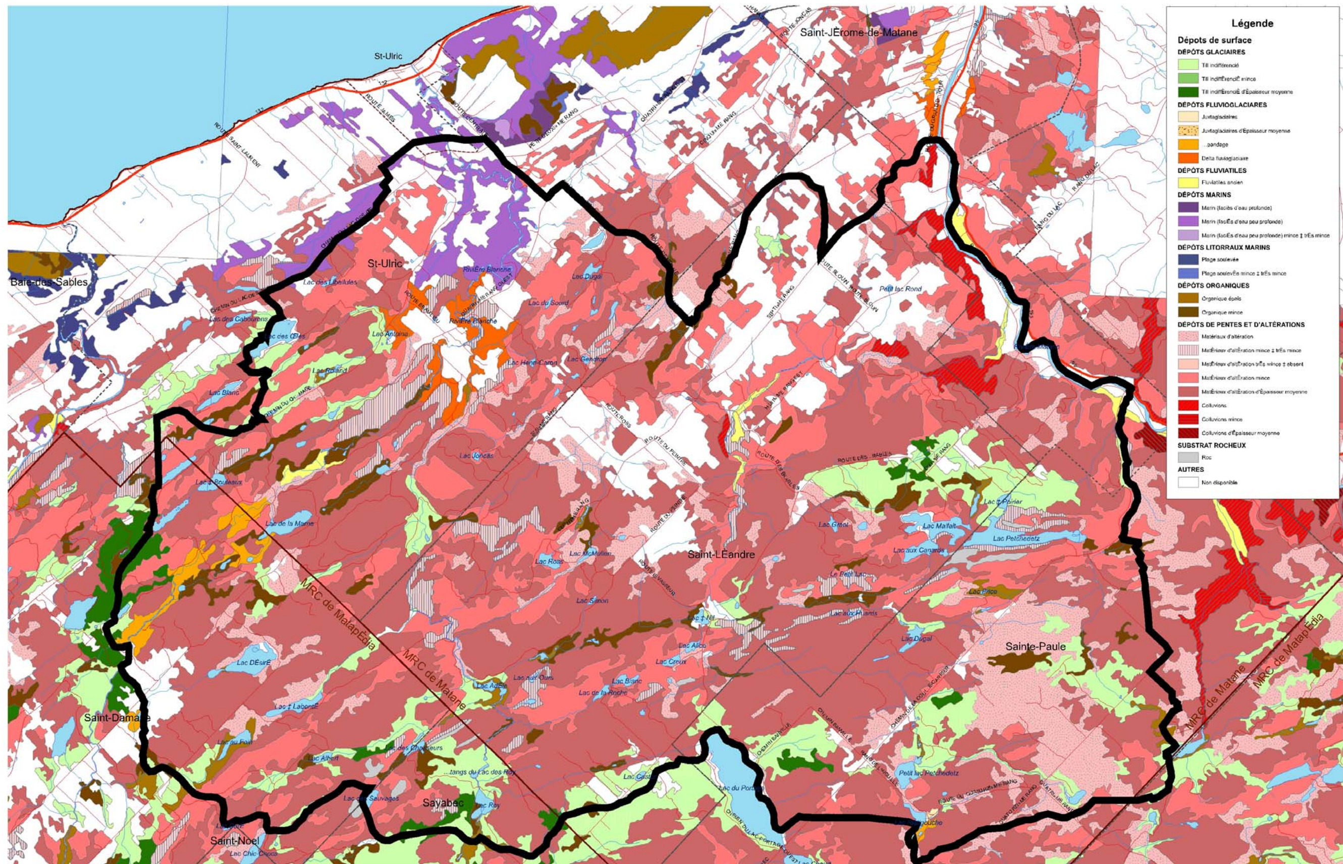
Figure 4 Dépôts meubles constituant la zone à l'étude (trait noir) (SNC-Lavalin inc. 2004)
