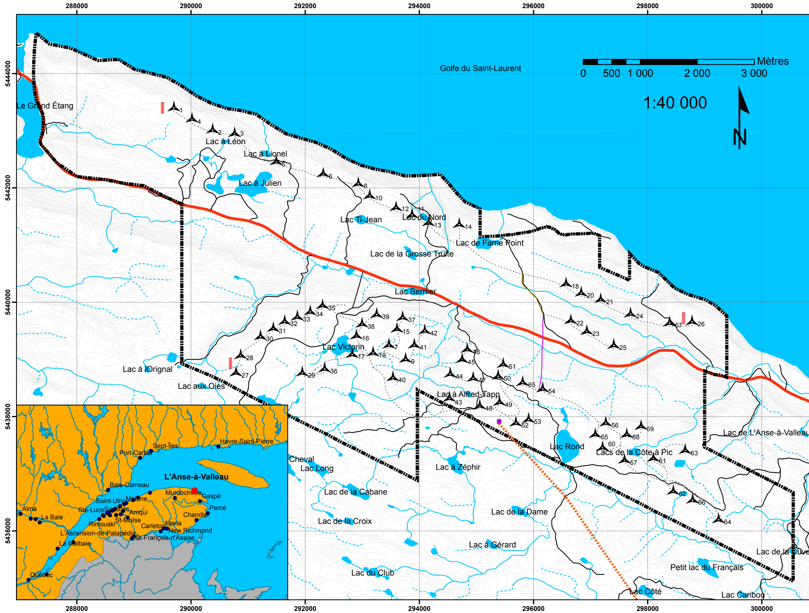
Carte 2.2 Positionnement des éoliennes dans le domaine du parc
