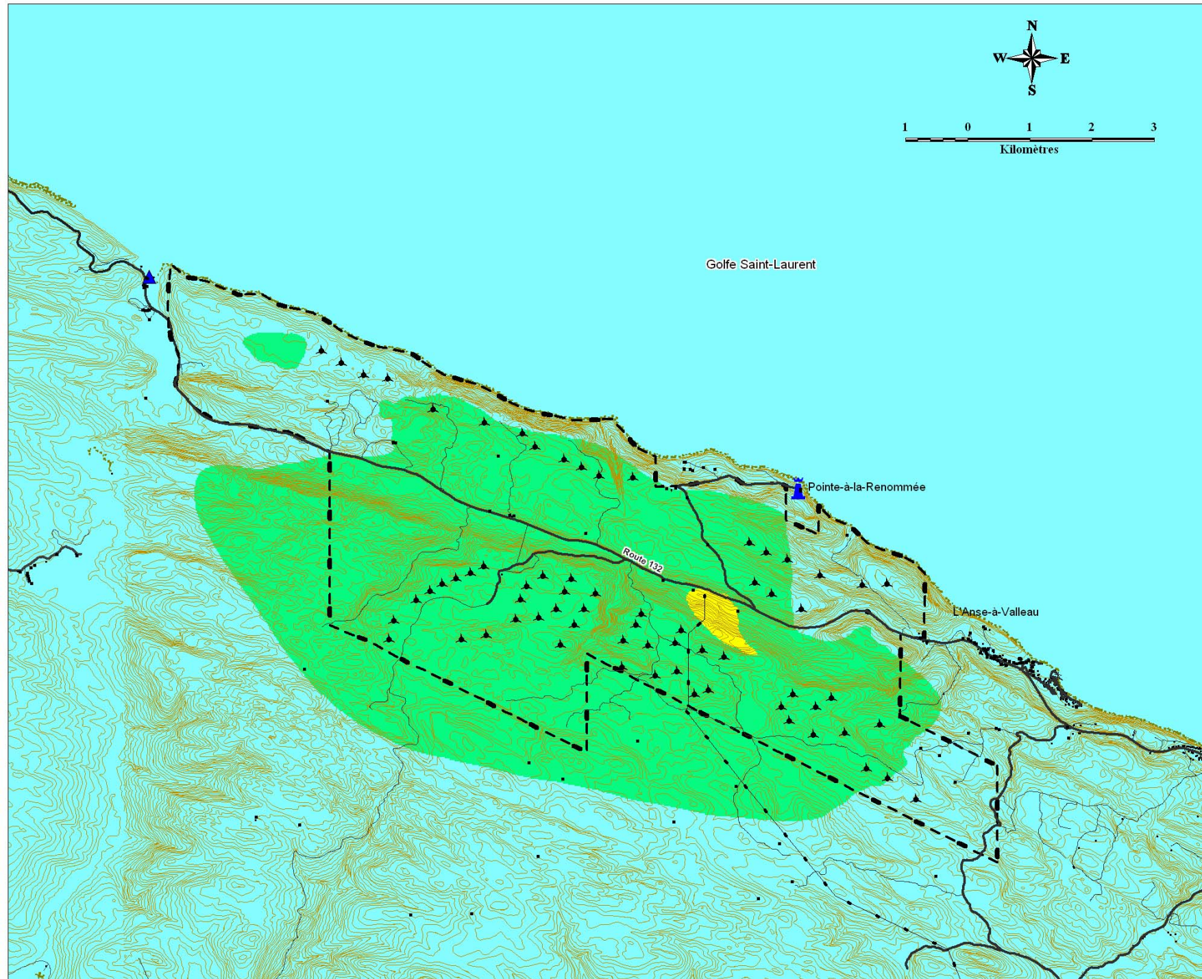
Carte 3 Prévision du brouillage par fantômes (CBGAT-22) (Avril 2005)
