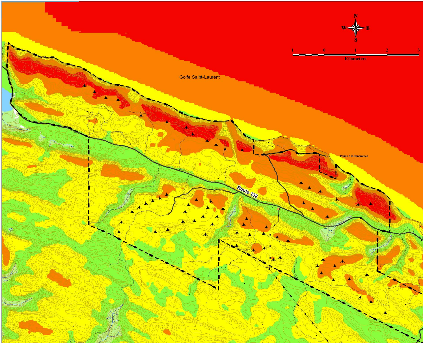
Carte 3.2 Qualité du gisement éolien (Avril 2005)
