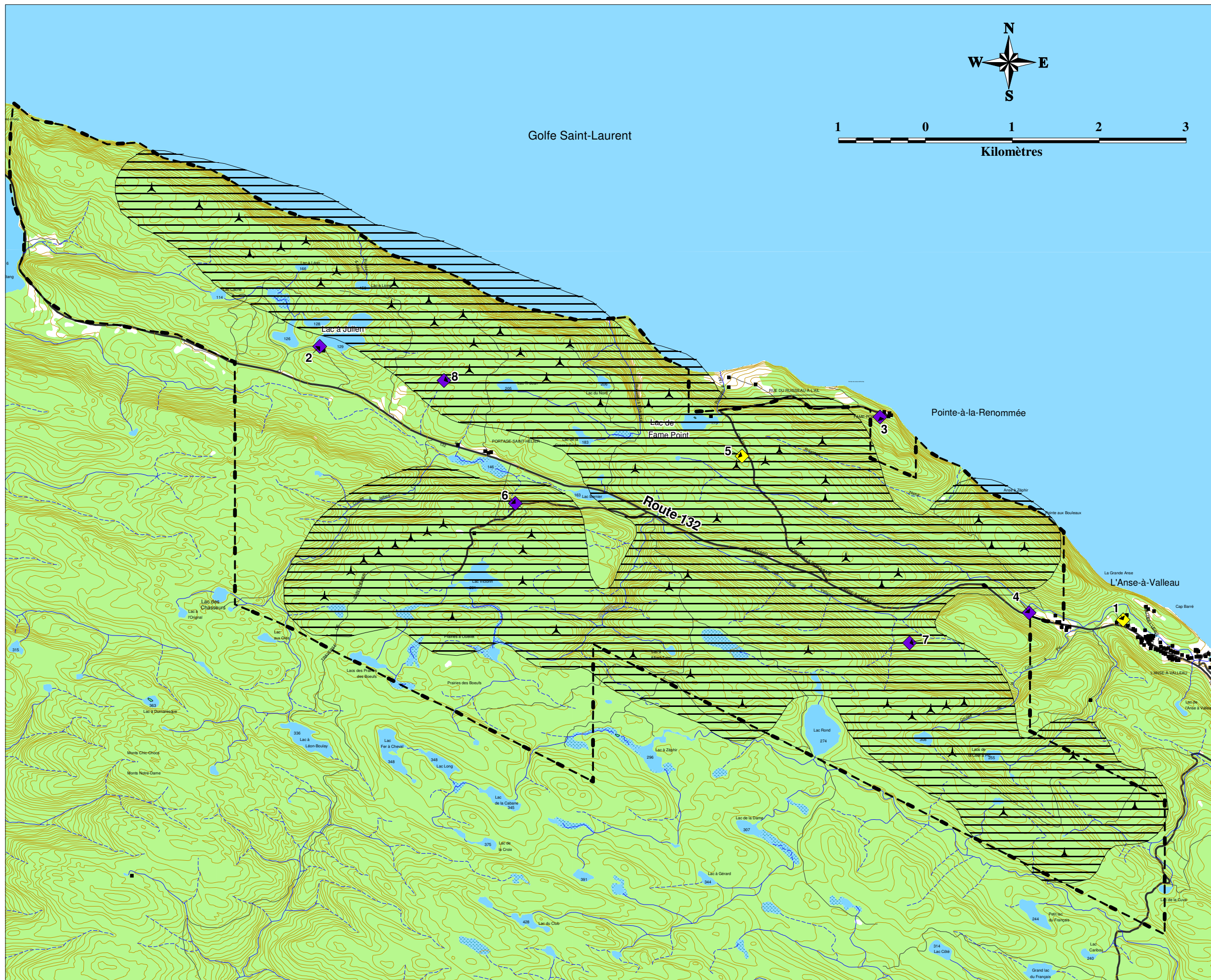
Carte 5.1 Contour isophonique du parc éolien (42 dBA)
